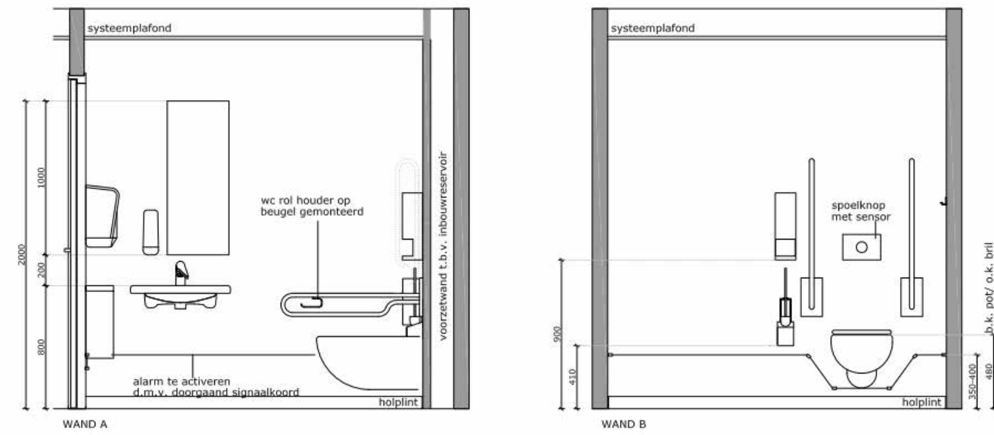
Indeling/aanzichten Miva toilet
