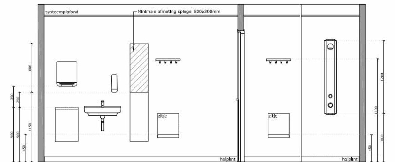
Indeling/aanzichten kleedruimte en douche
