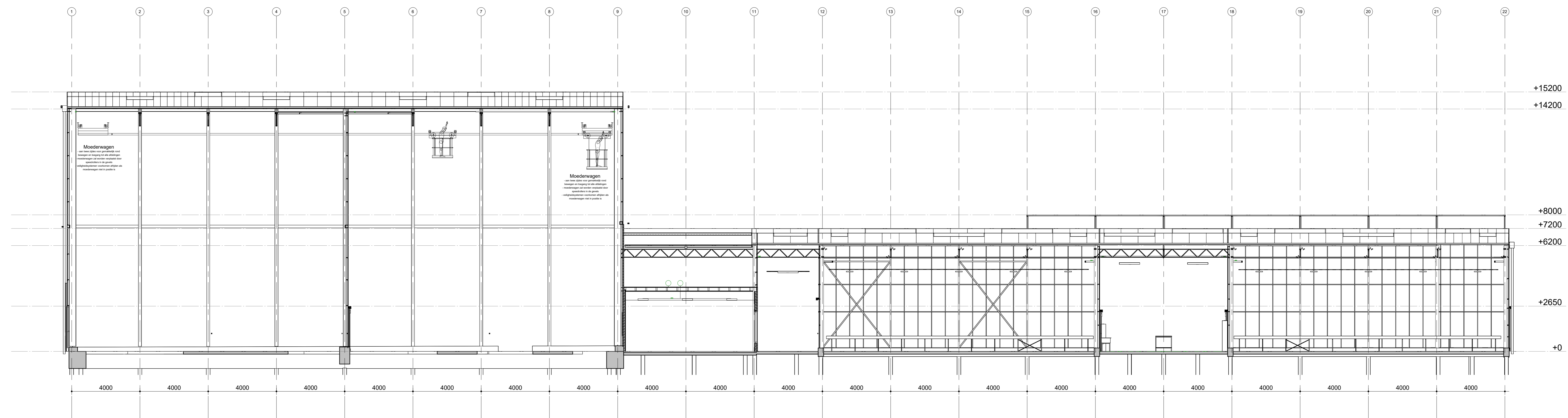
Doorsnede F 1 : 100
