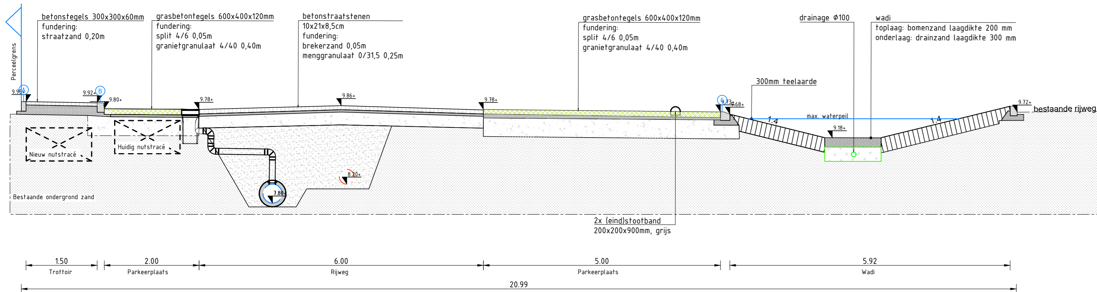
Doorsnede A-A
