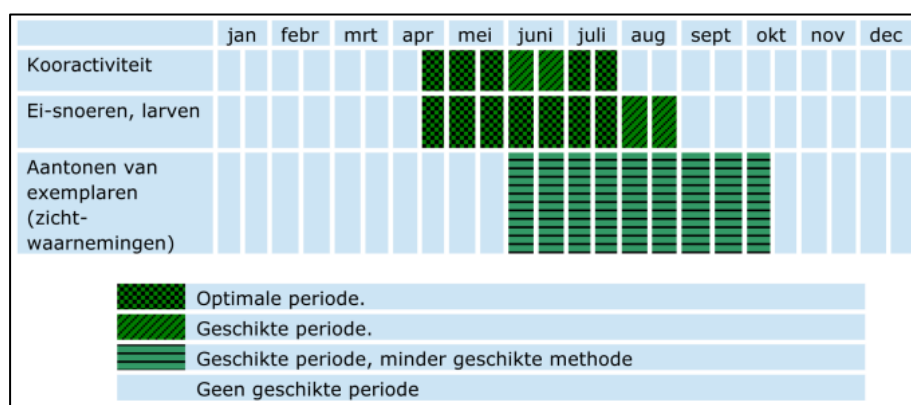
Afbeelding 1. Geschiktheid van inventarisatieperioden voor verschillende methoden van inventariseren van de Rugstreeppad (BIJ12).
