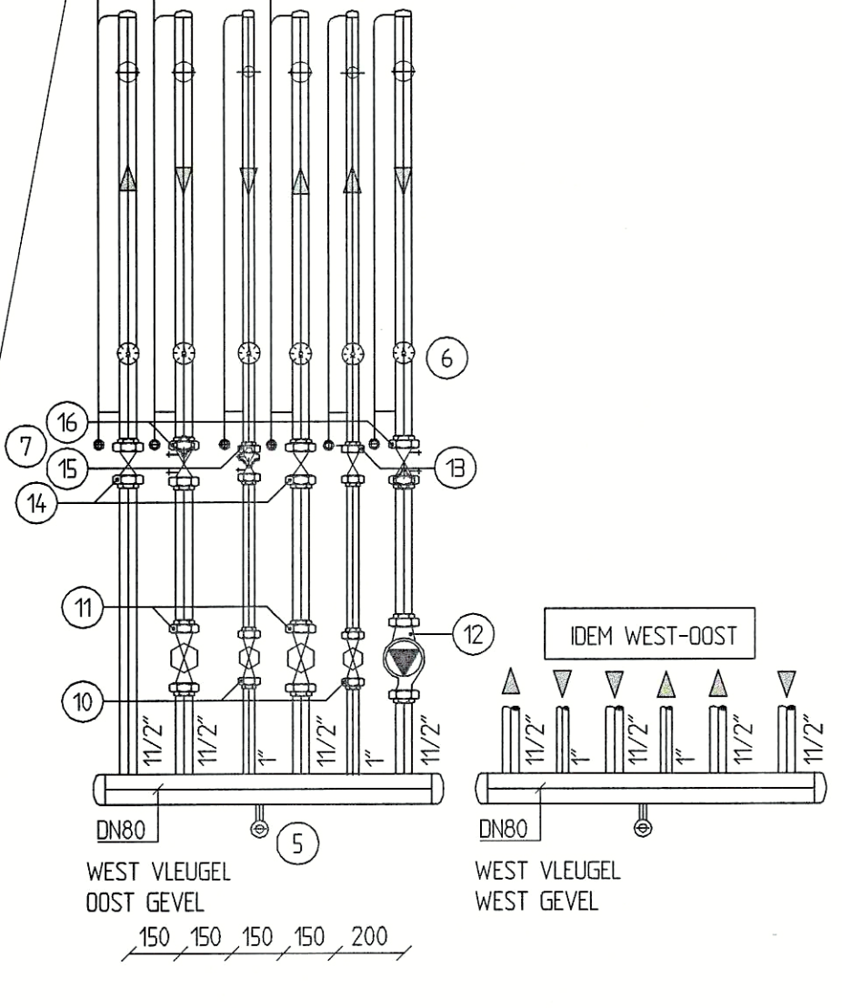
AANZICHT B
