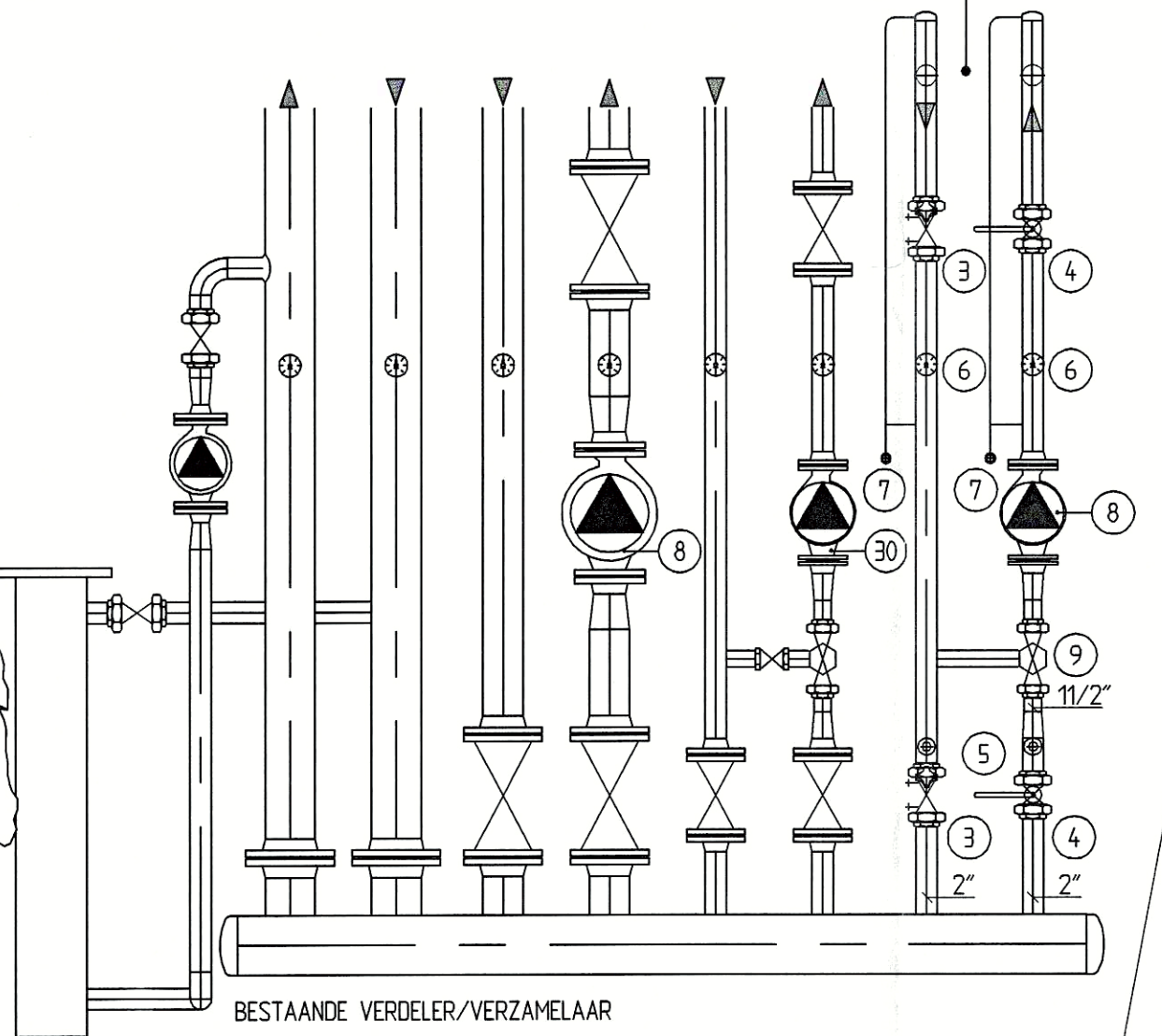
AANZICHT A
