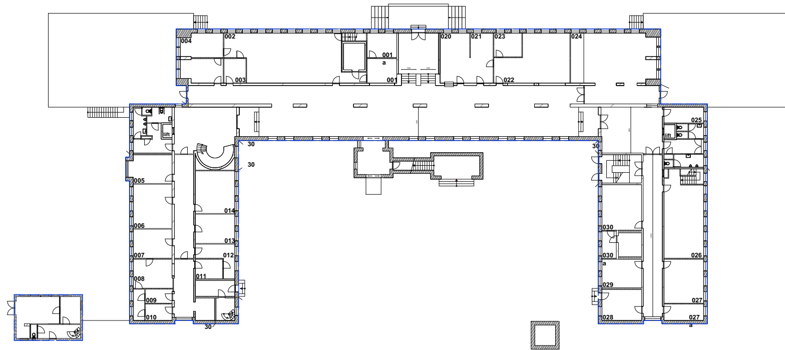
begane grond | bvo: 1696 m 2 + 54 m 2 (excl. toren) ---
