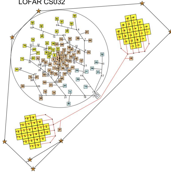
LOFAR CS032
