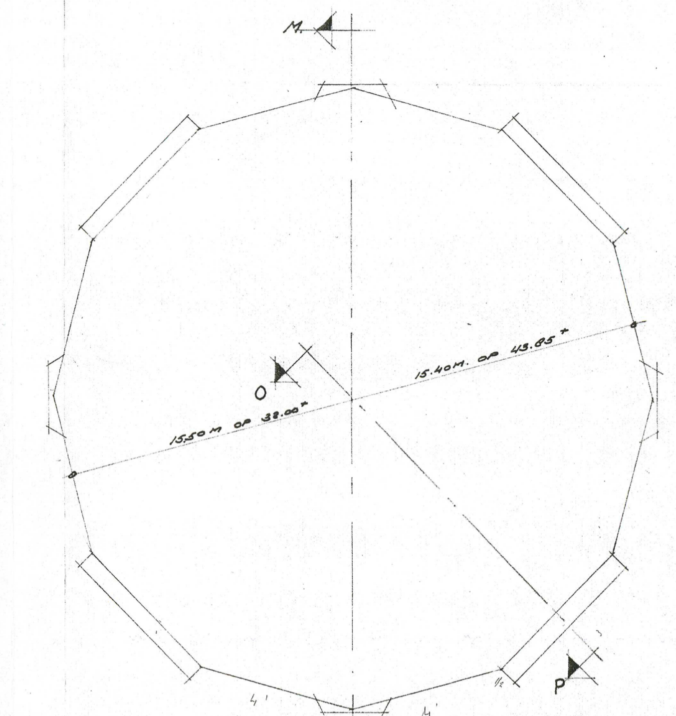
DOORSNEDEN G-H.
