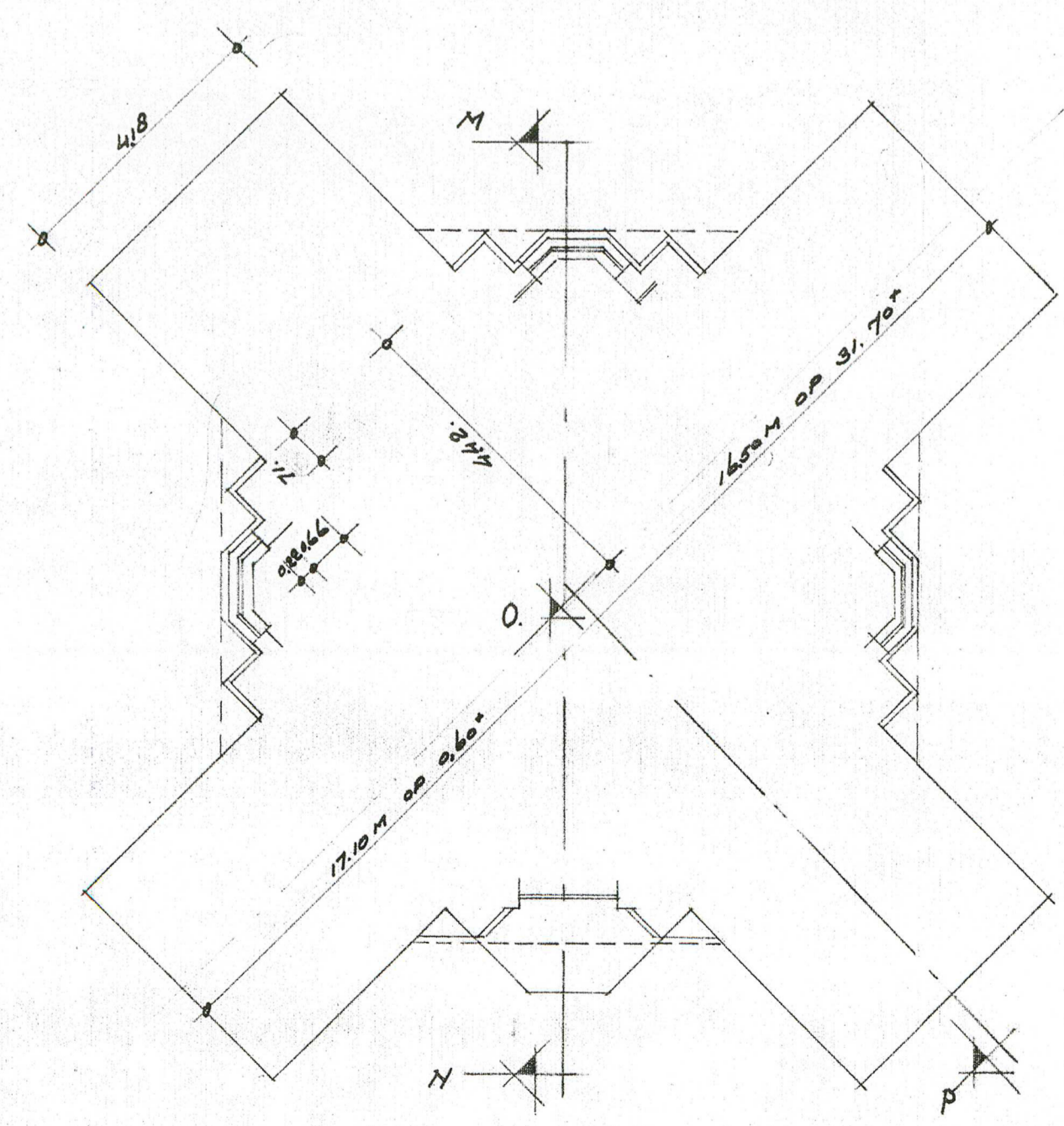
DOORSNEDEN A-B.
