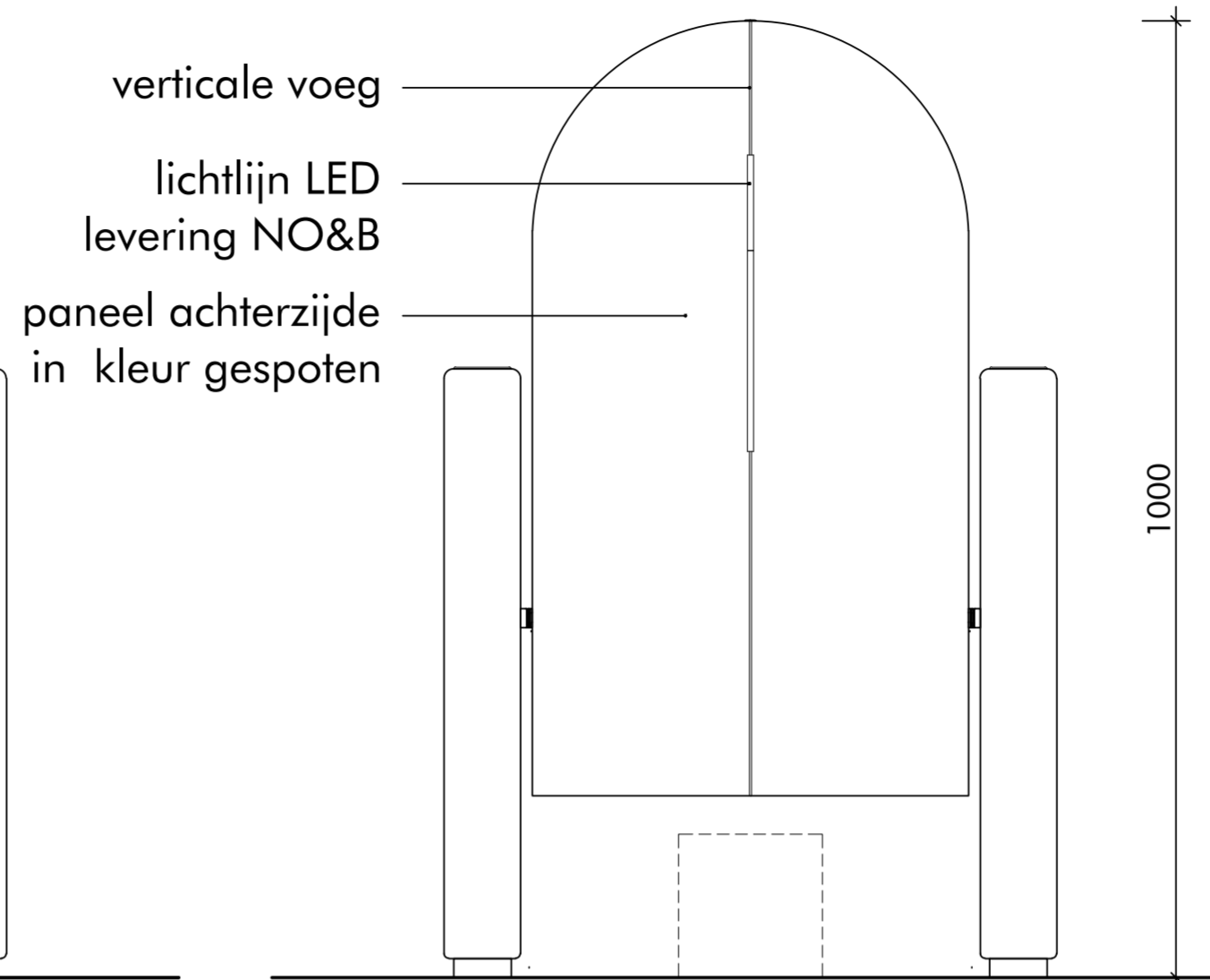
aanzicht achterzijde
