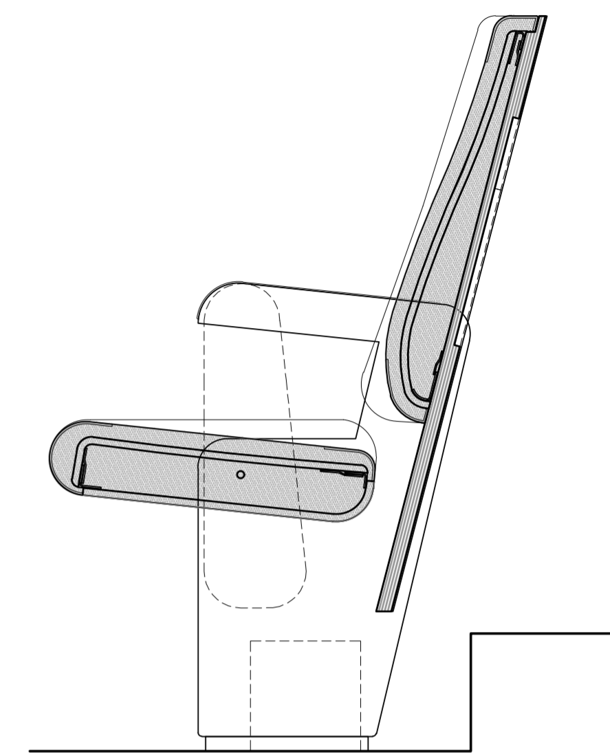
doorsnede
