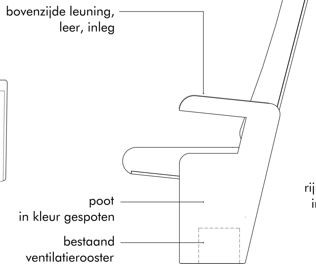
zijaanzicht
