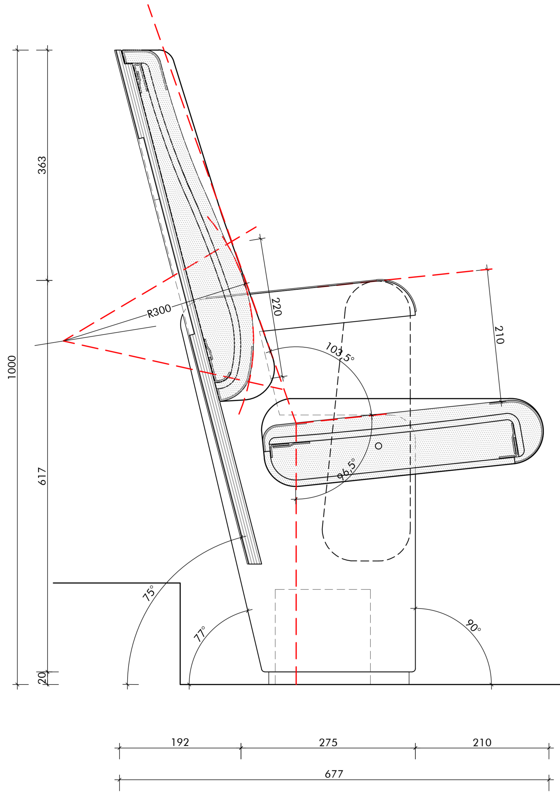
doorsnede
