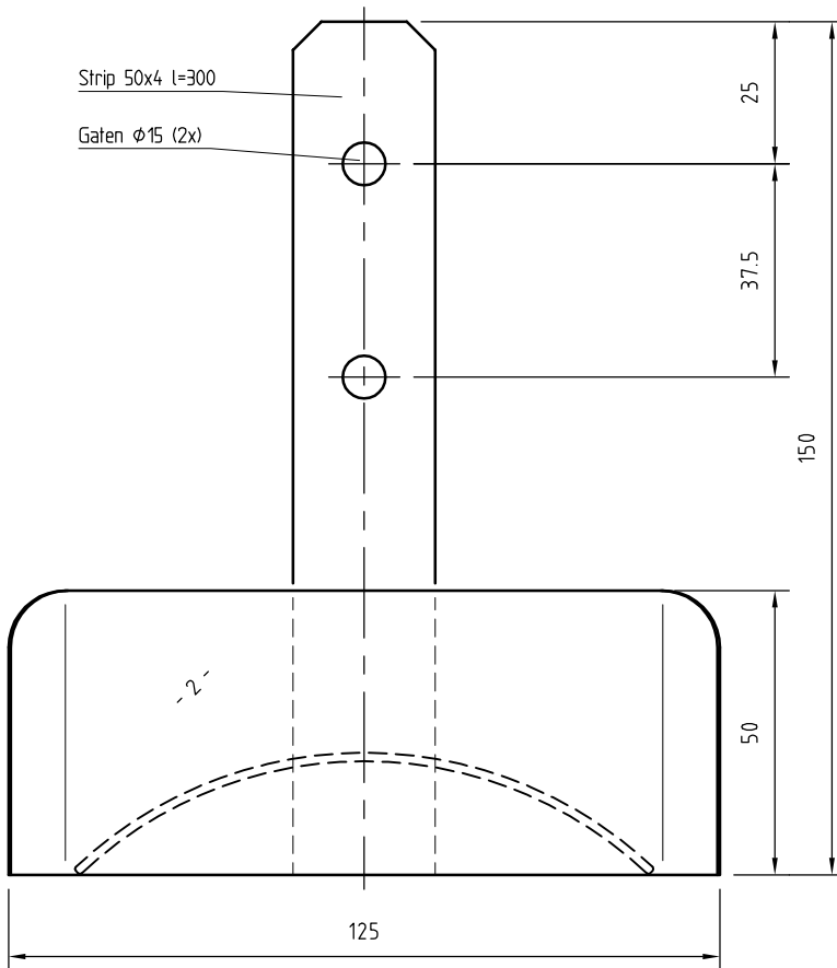
Vooraanzicht
