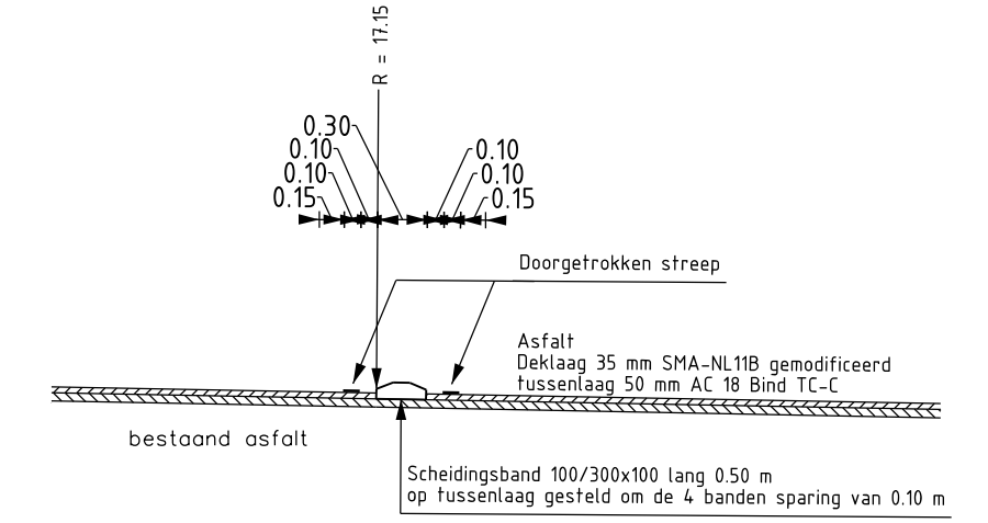
DOORSNEDE ROTONDE GELEIDEBAND BIJ AANBRENGEN DEKLAAG EN TUSSENLAAG schaal 1:50
