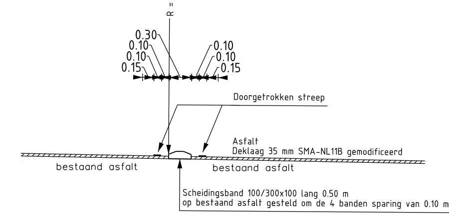
DOORSNEDE ROTONDE GELEIDEBAND BIJ AANBRENGEN DEKLAAG schaal 1:50
