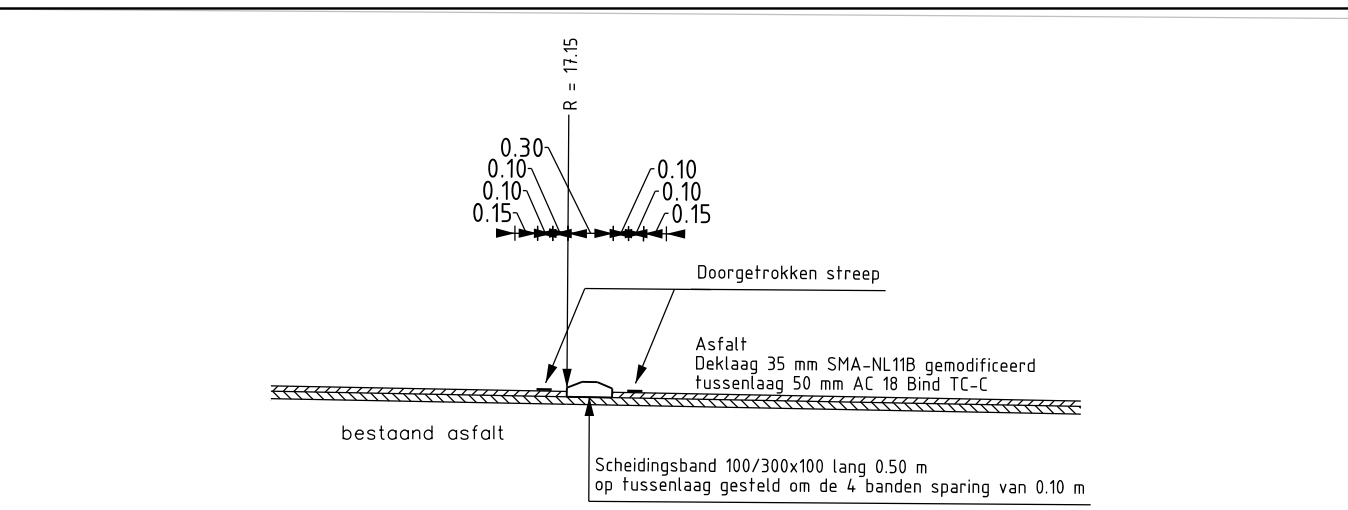
DOORSNEDEN ROTONDE GELEIDEBAND BIJ AANBRENGEN DEKLAAG EN TUSSENLAAG Schaal 1:50
