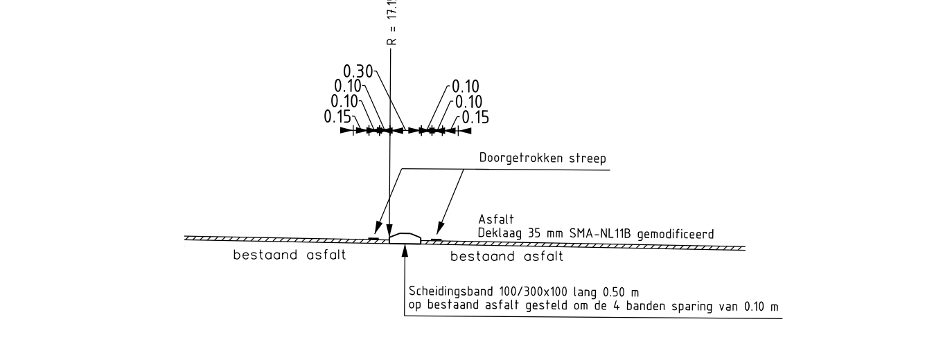
DOORSNEDEN ROTONDE GELEIDEBAND BIJ AANBRENGEN DEKLAAG Schaal 1:50
