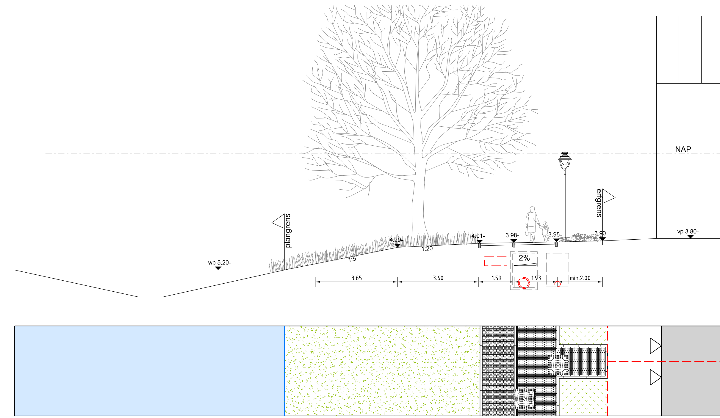
Profiel 10
