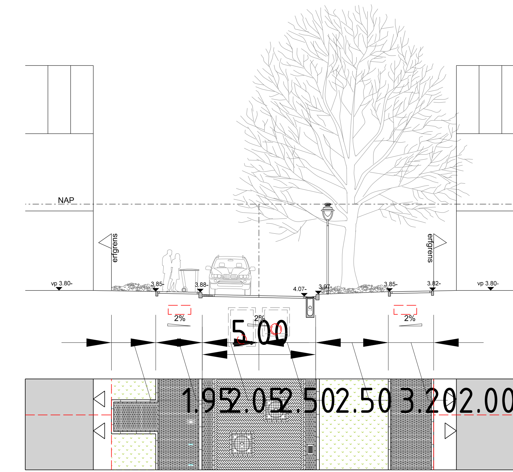
Profiel 11
