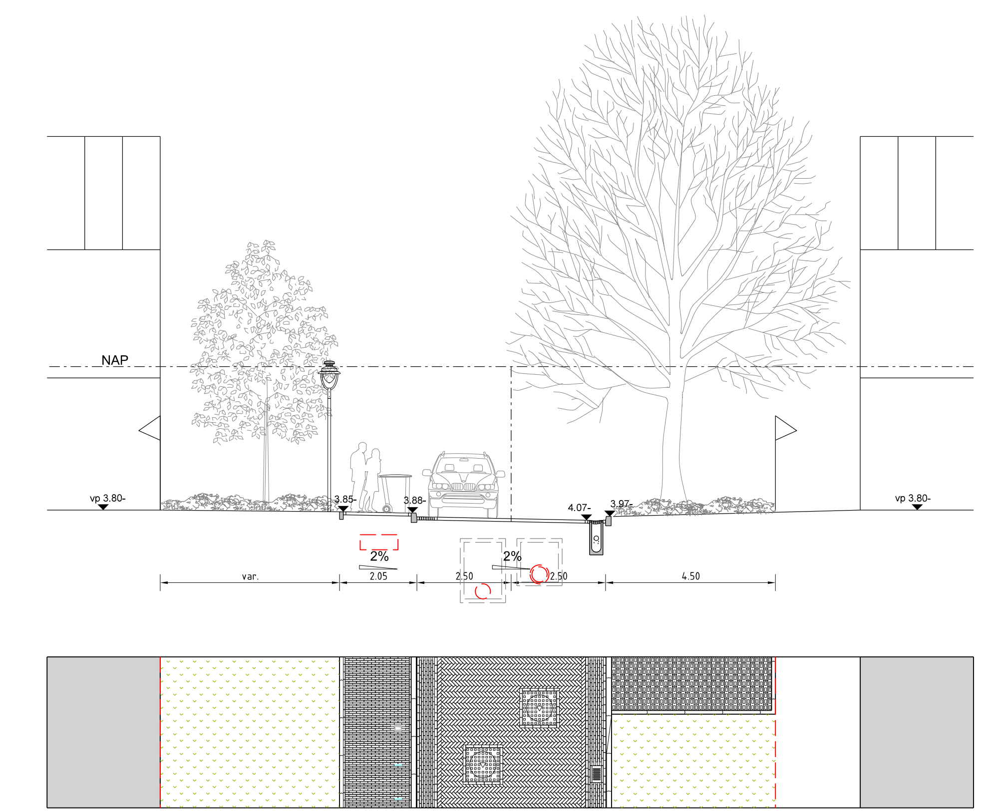
Profiel 16
