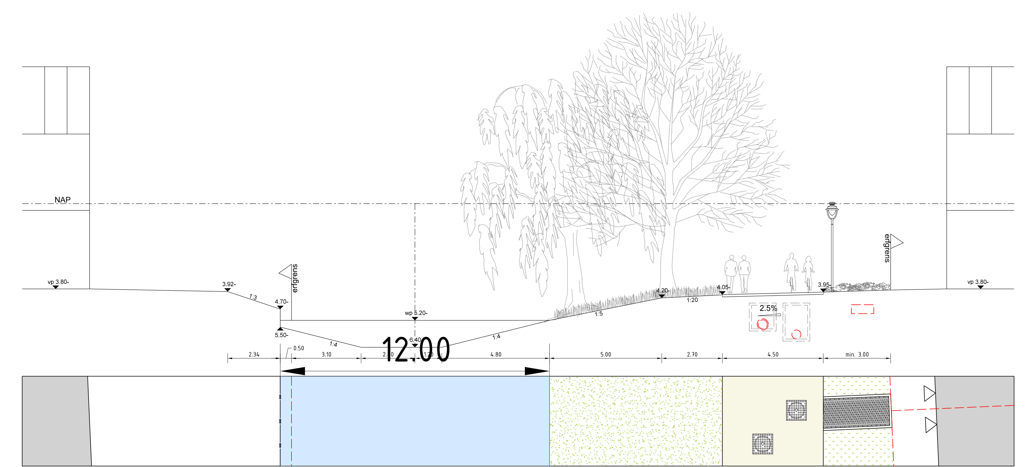
Profiel 13 rechts
