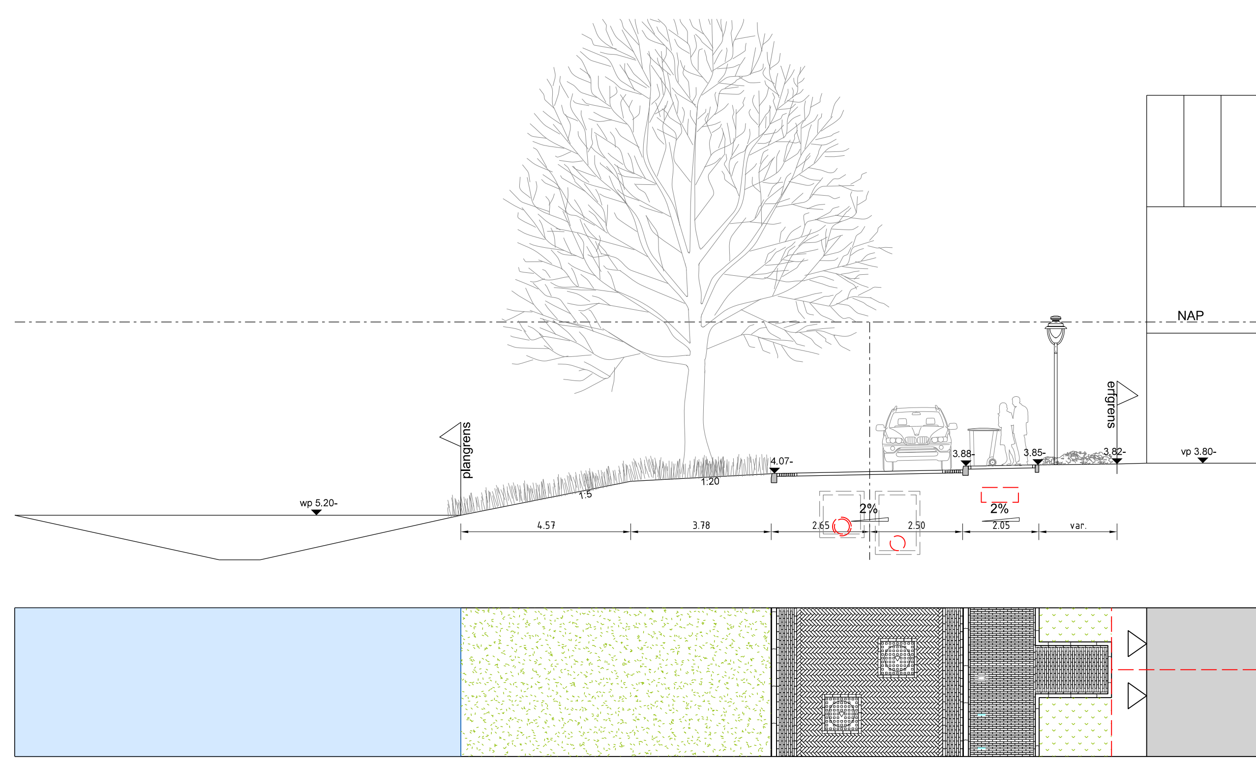
Profiel 9
