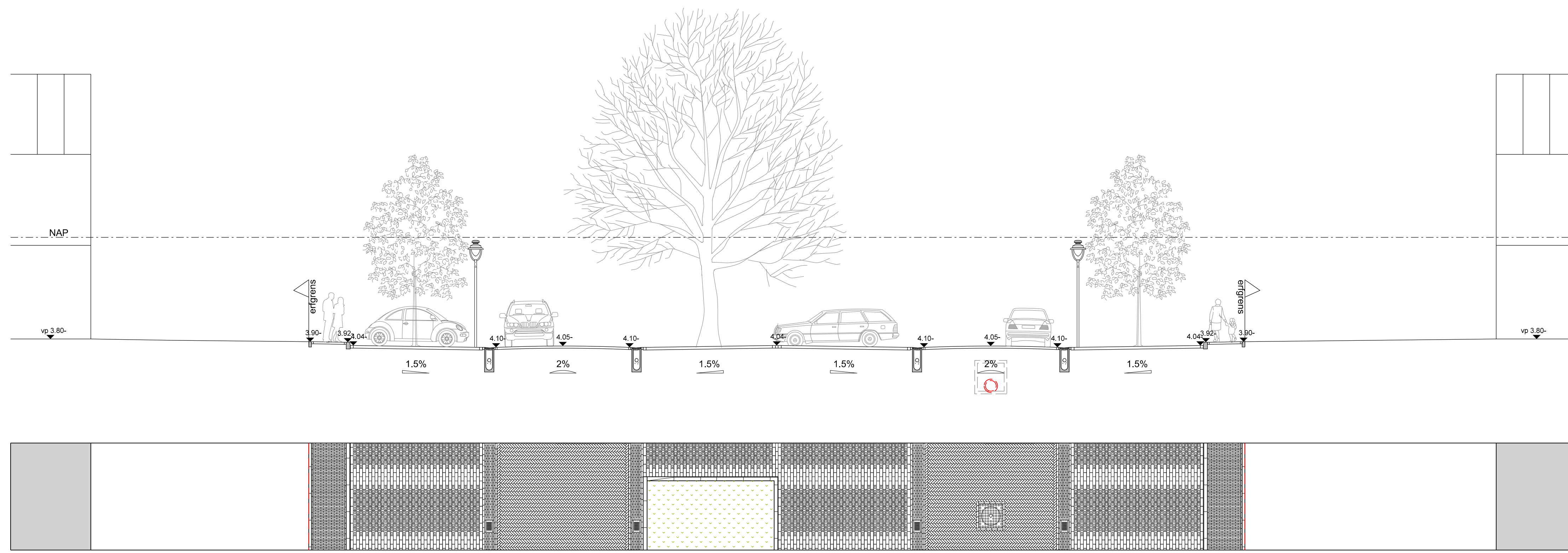
Profiel 14
