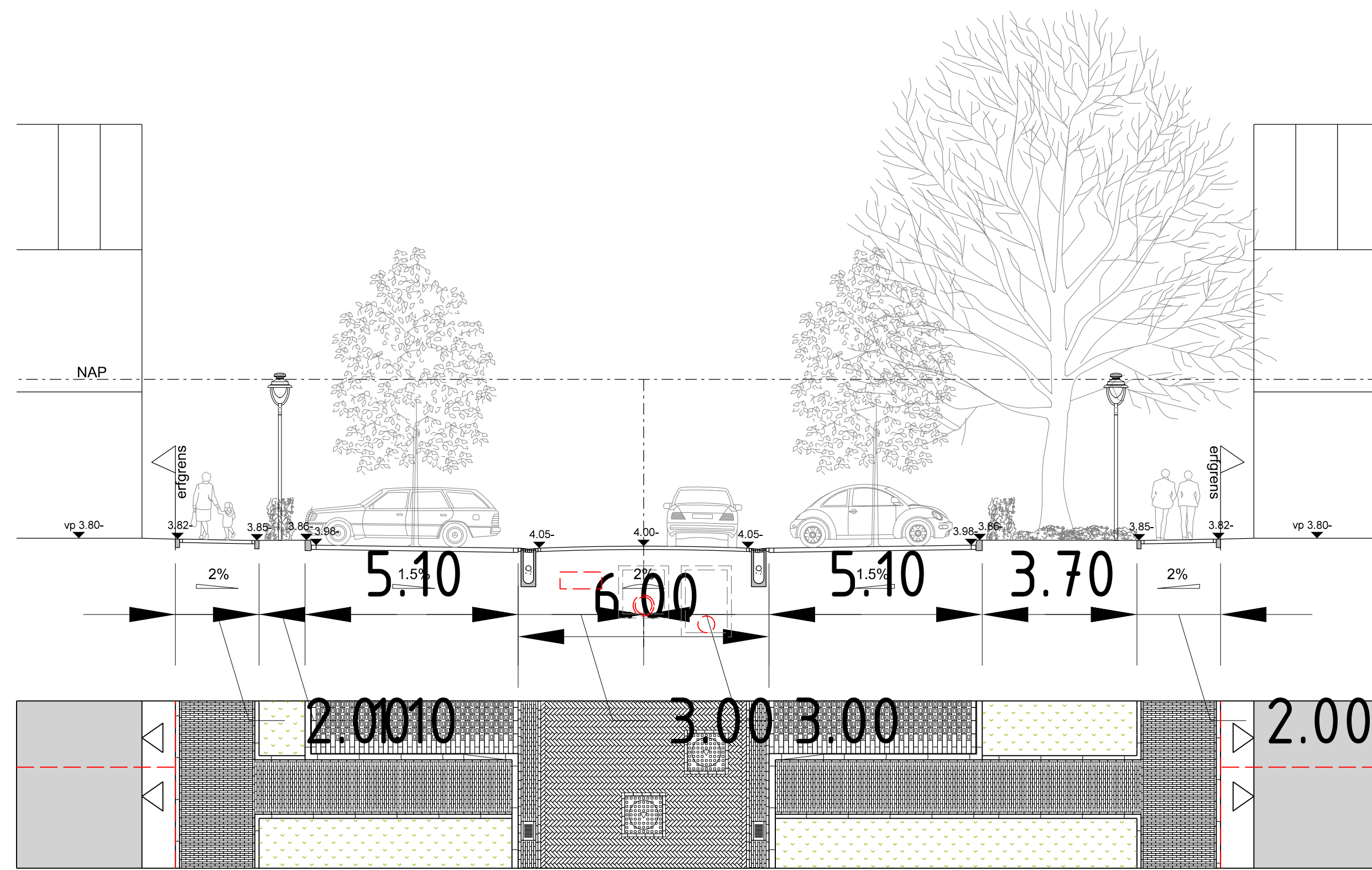
Profiel 12
