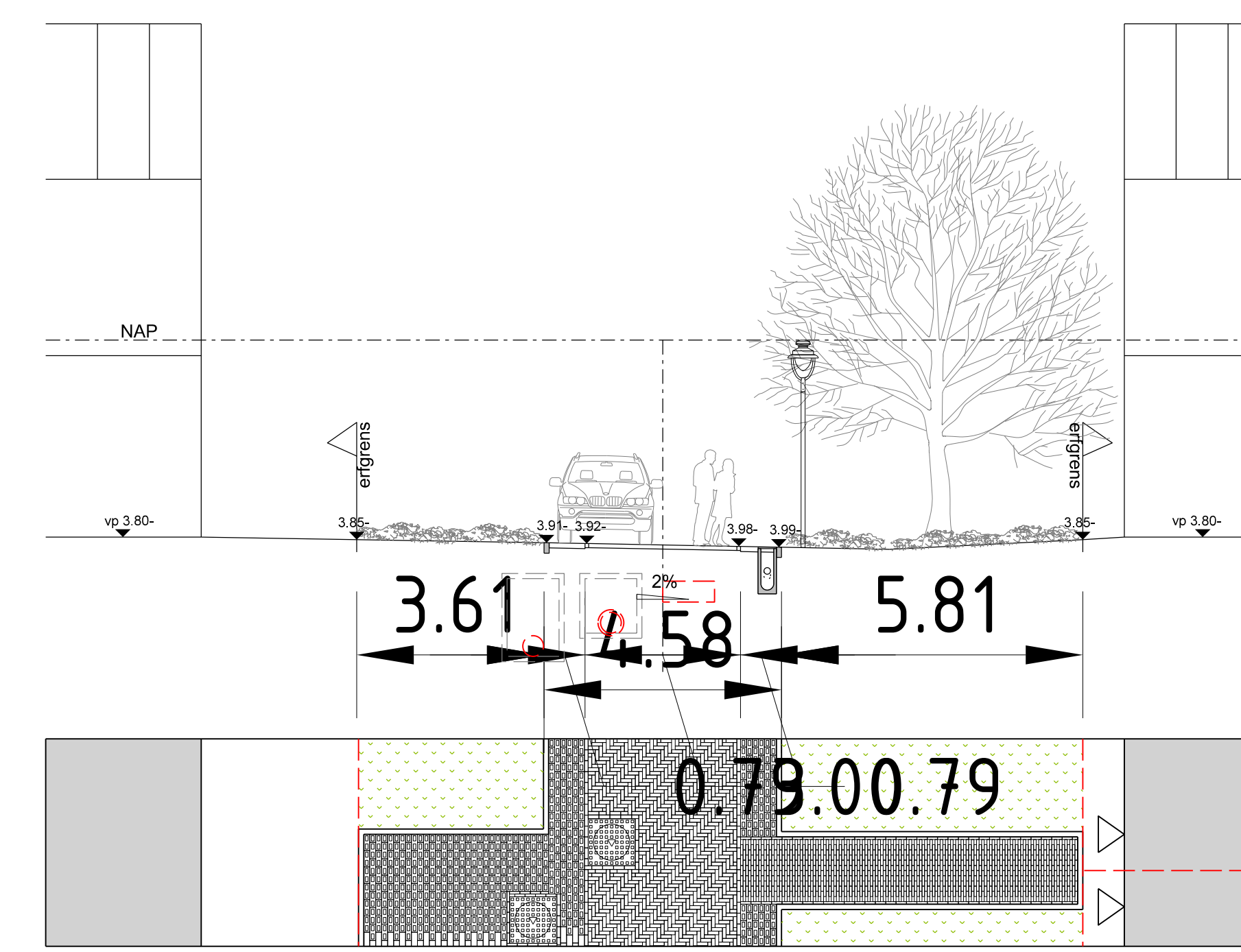
Profiel 15
