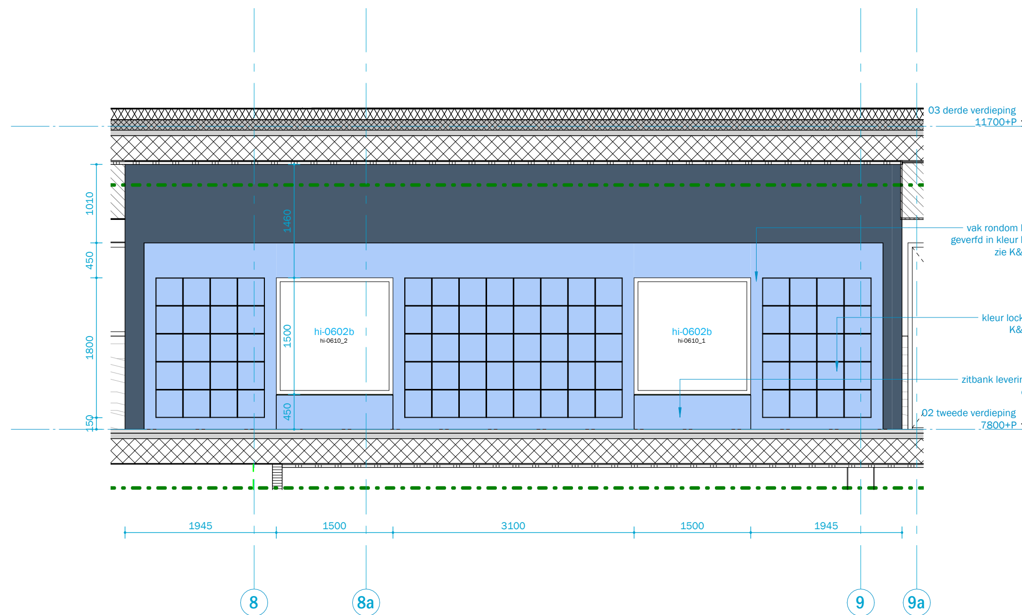
Doorsnede C
