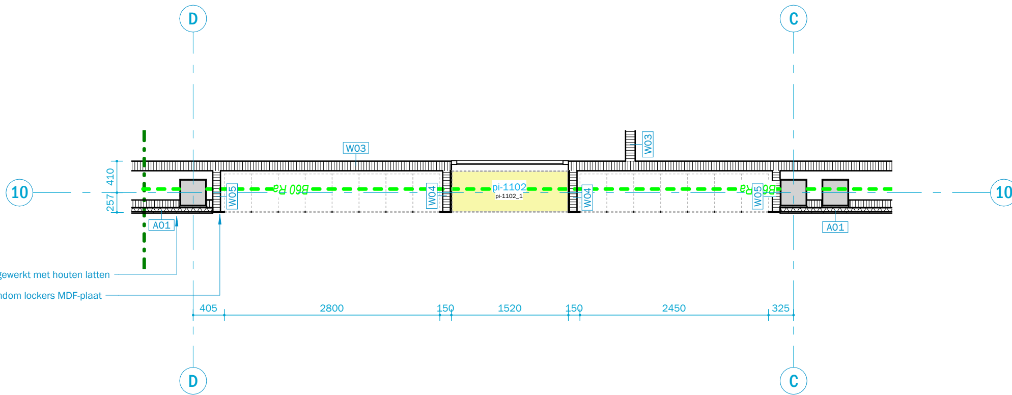
Uitsnede plattegrond
