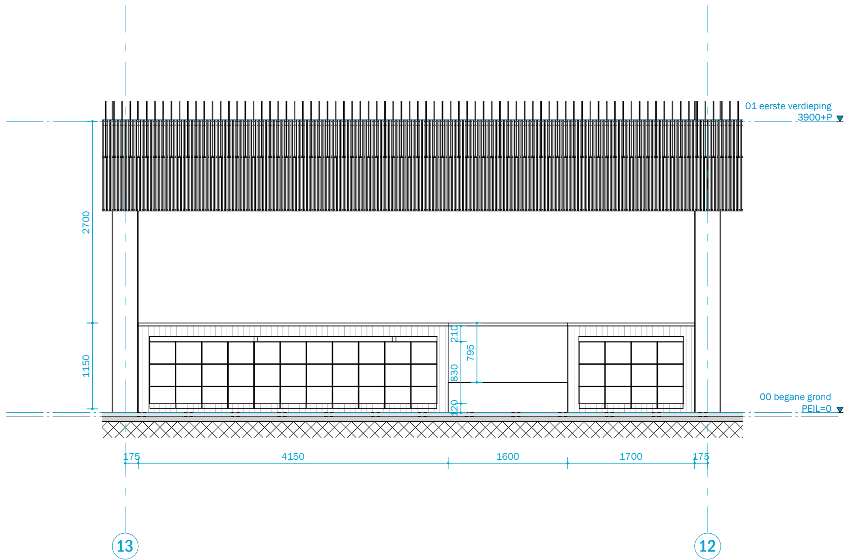
Doorsnede A
