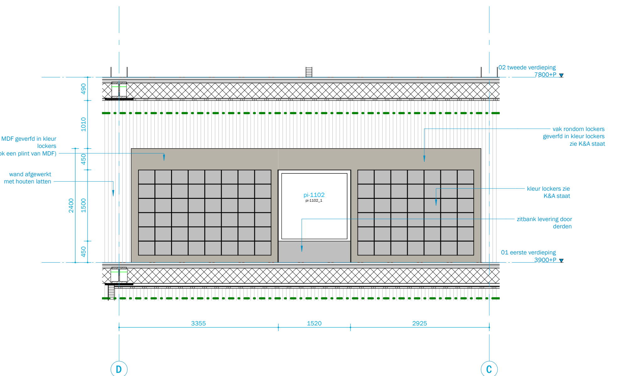
Doorsnede B
