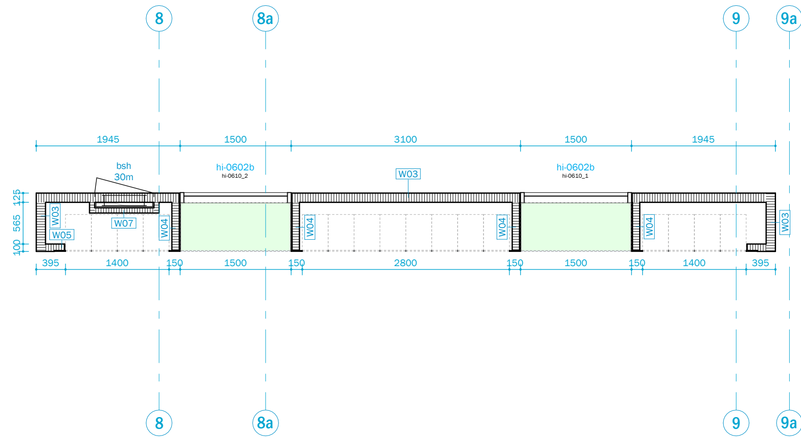
Uitsnede plattegrond lockers V2
