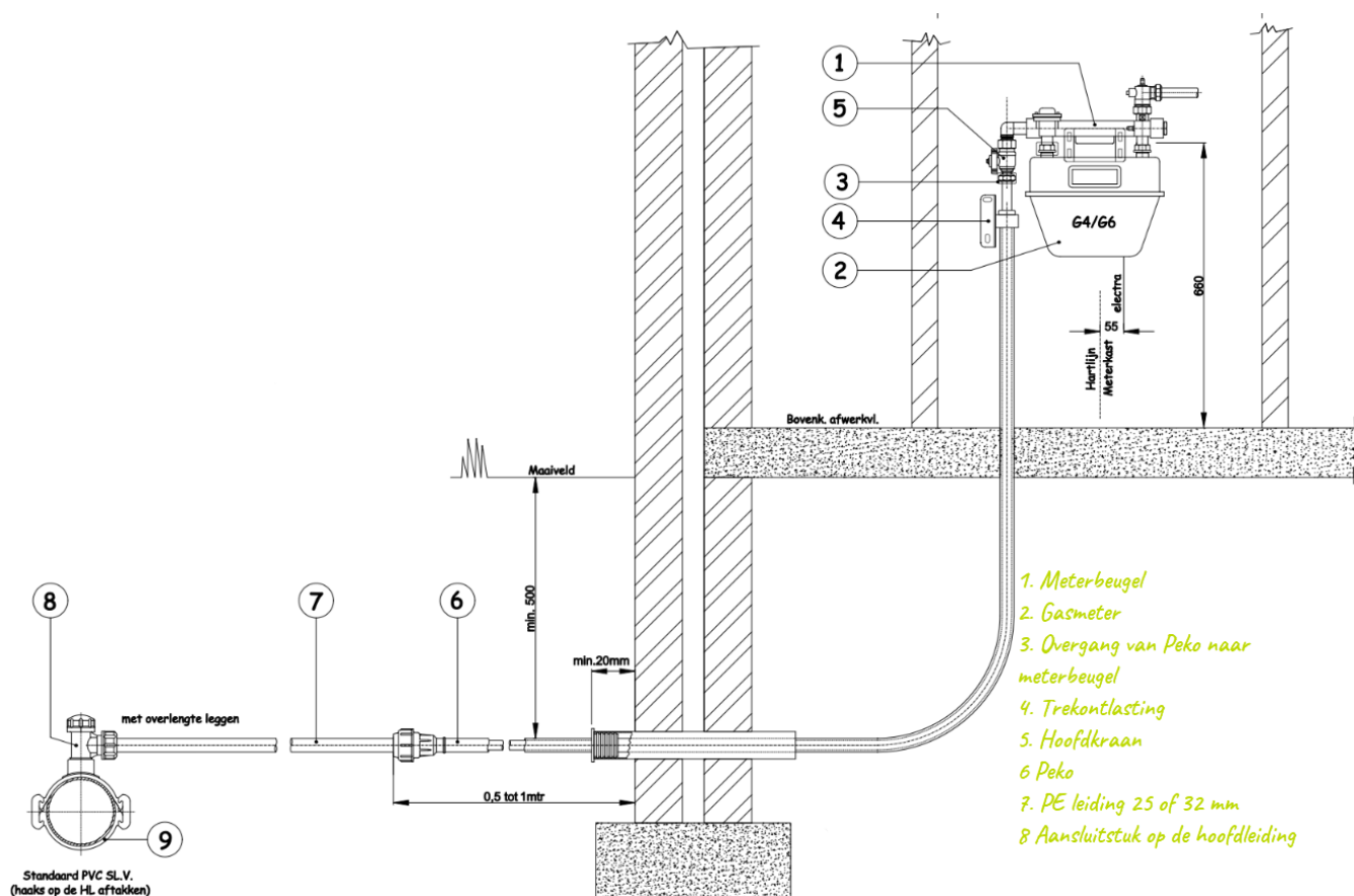
Figuur 1 Situatieschets saneringsconstructie
