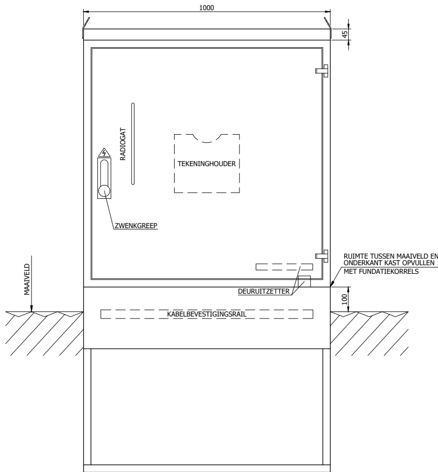
VOORAANZICHT
