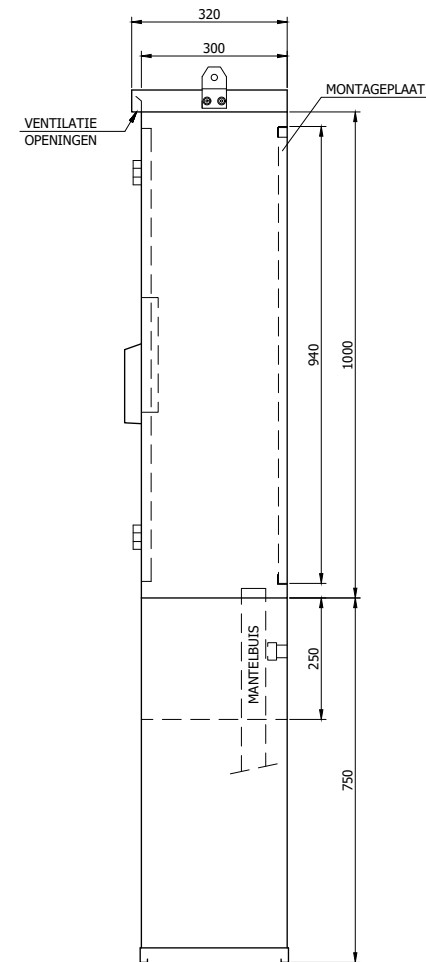
ZIJAANZICHT RECHTS
