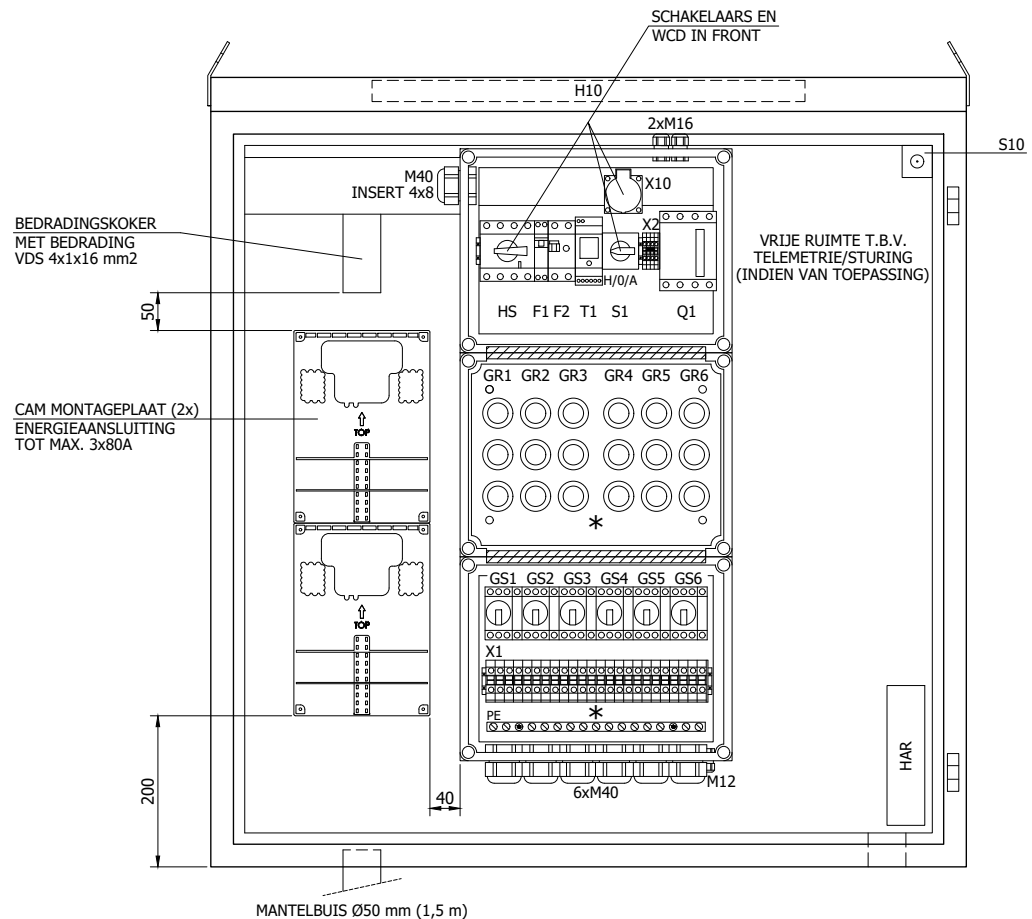
VOORAANZICHT (ZONDER DEUR EN SOKKEL)
