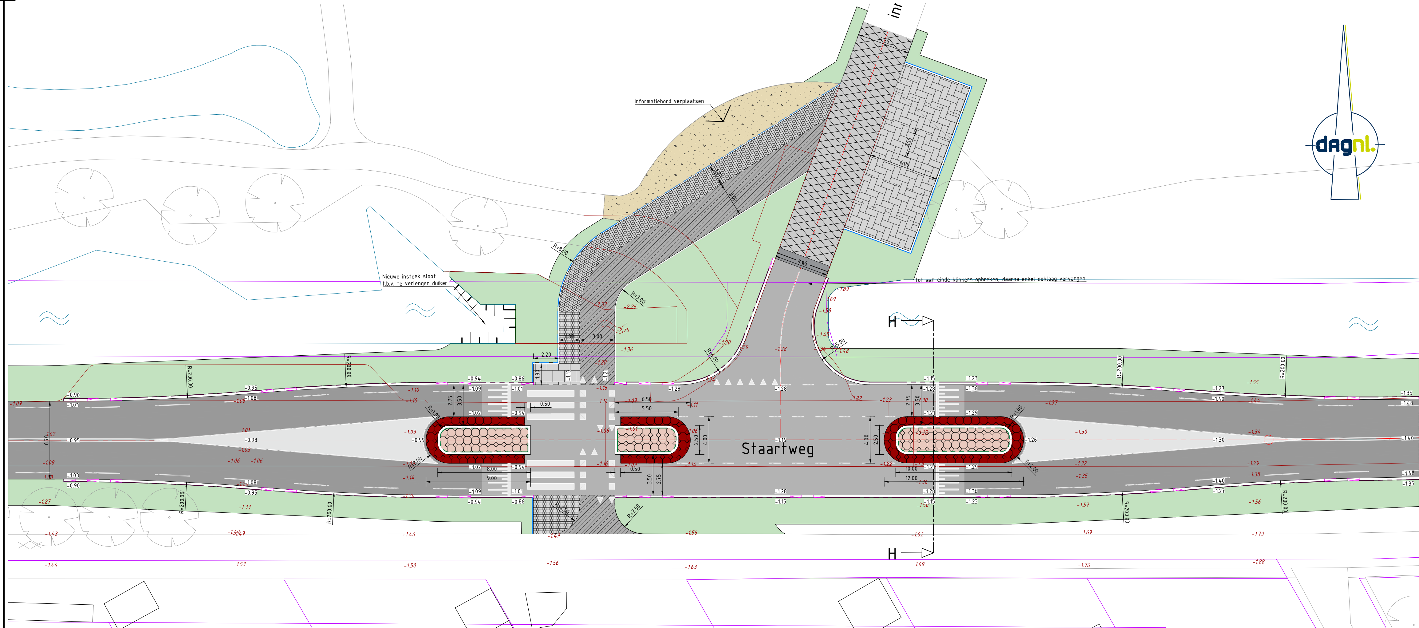
DEELSITUATIE 10 schaal 1:200
