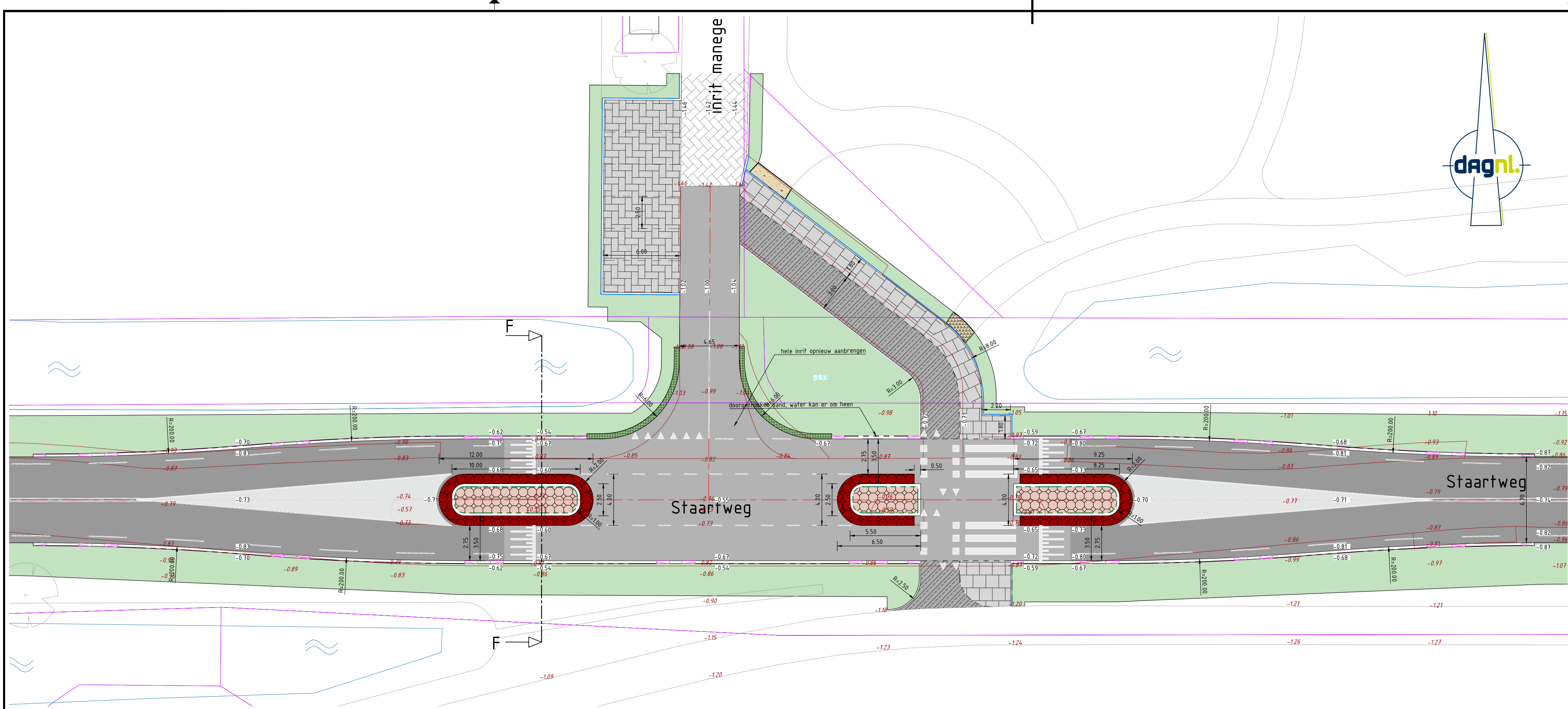
DEELSITUATIE 9 schaal 1:200
