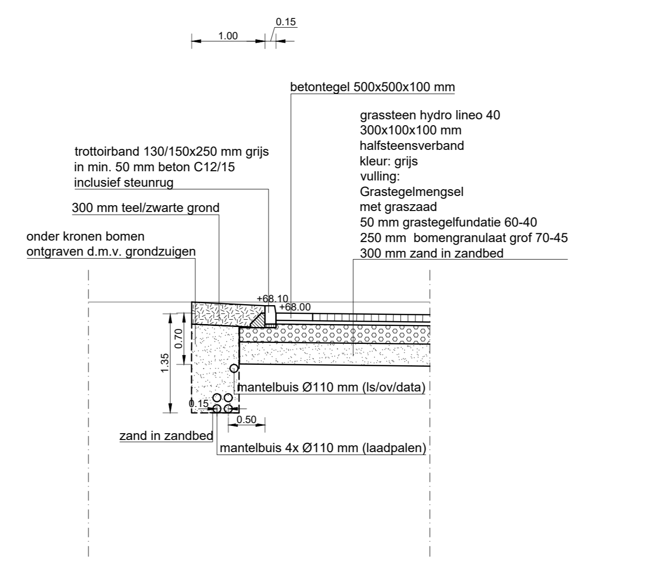
Dwarsprofiel V-V (mantelbuizen) schaal: 1:50
