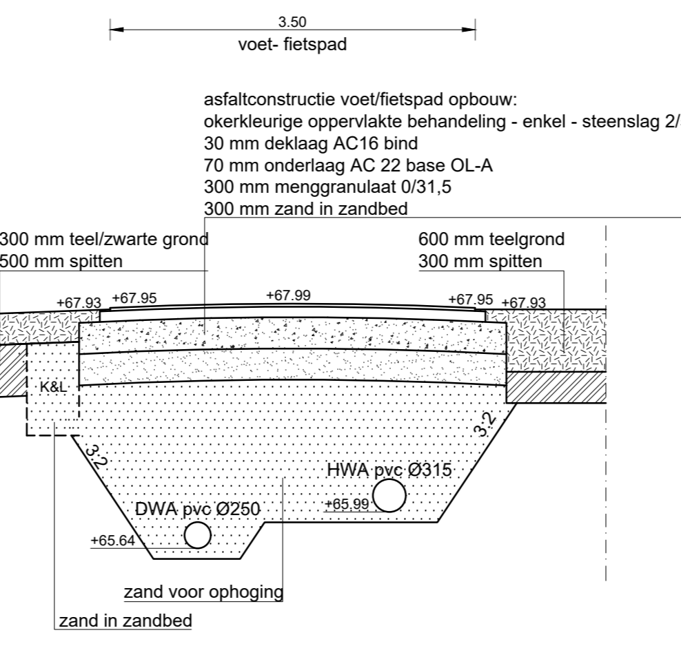
Dwarsprofiel W-W schaal: 1:50
