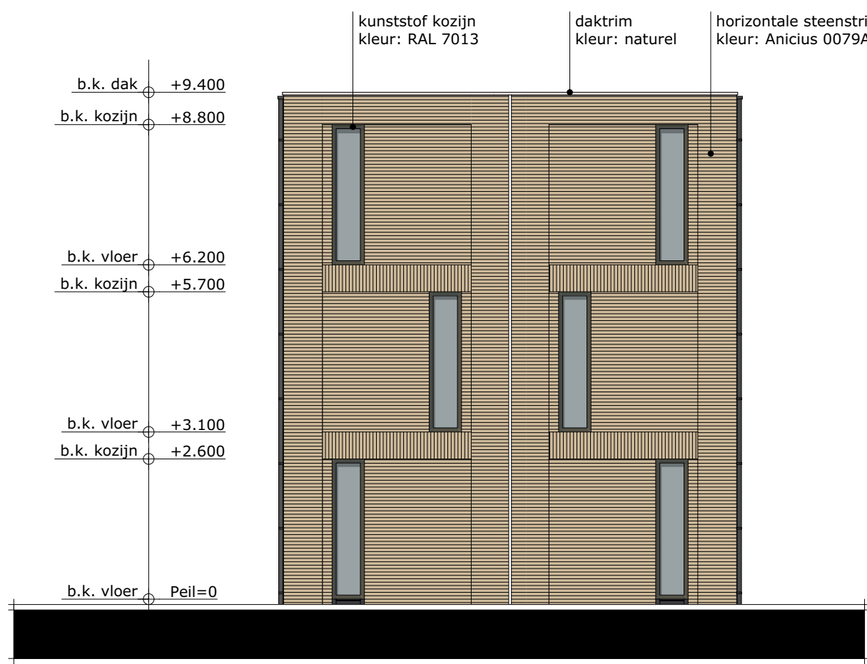
WESTGEVEL
