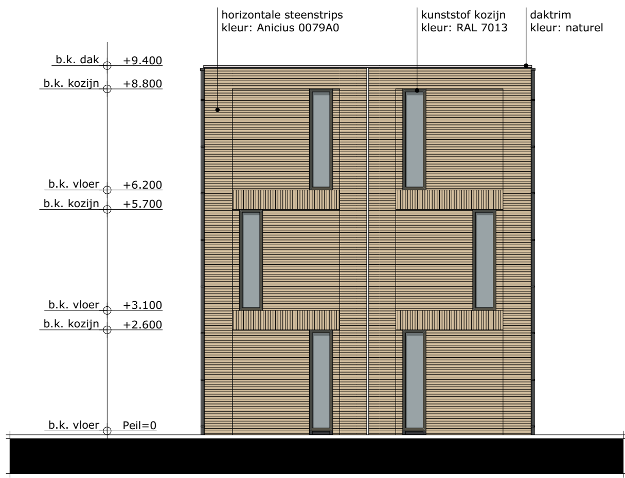
OOSTGEVEL
