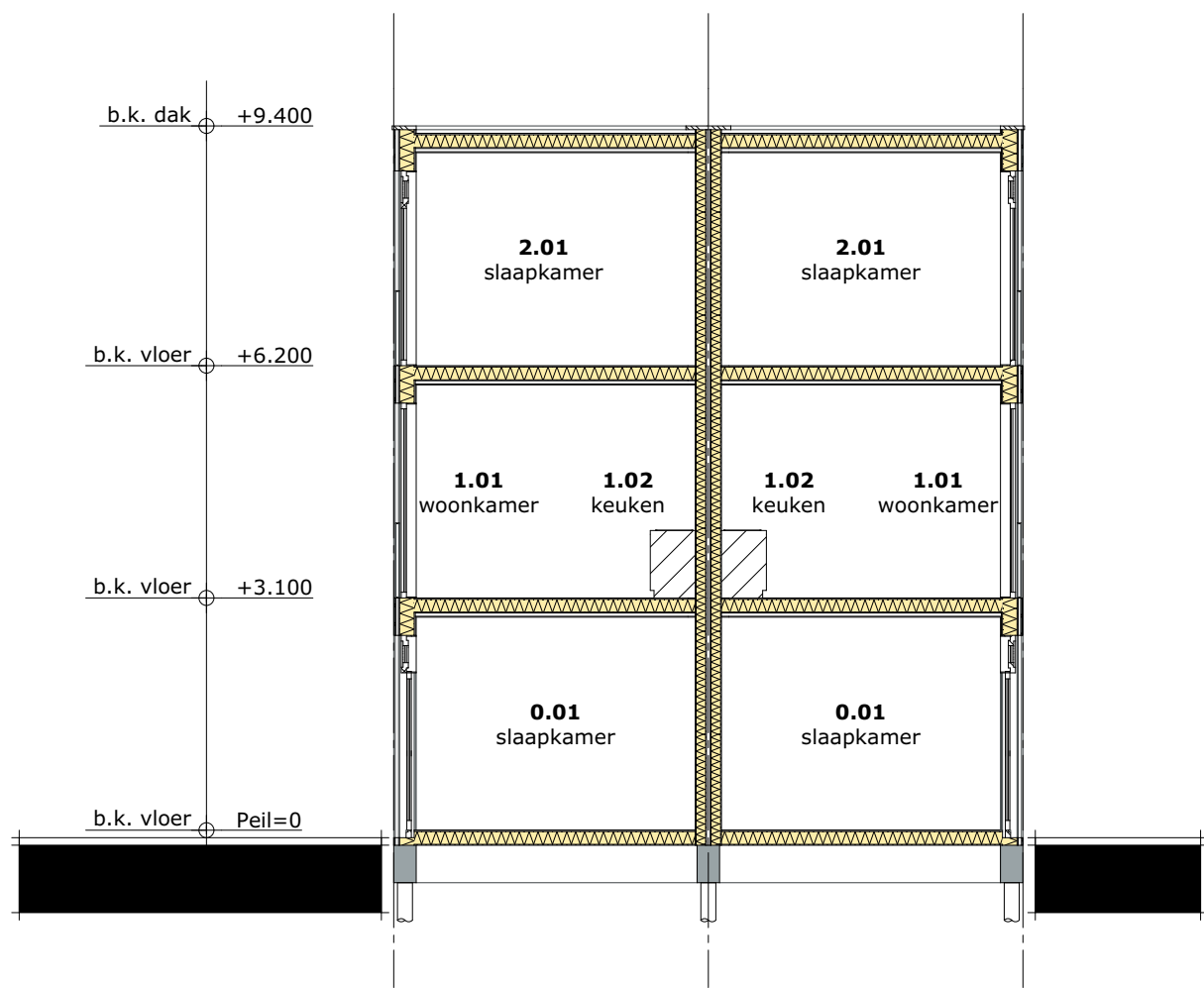
DOORSNEDE B-B
