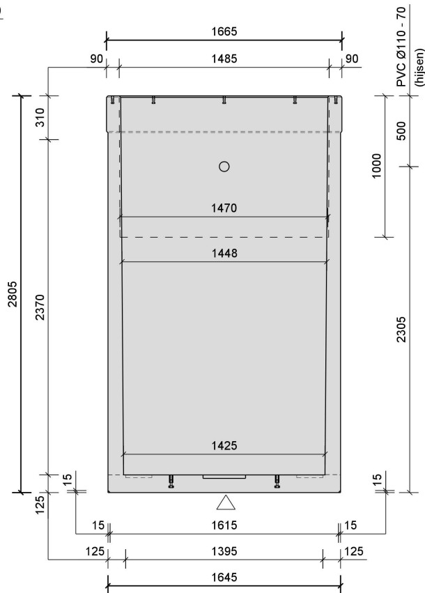
Doorsnede A 1:25
