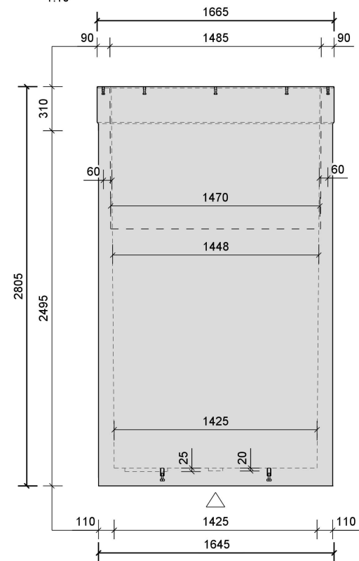
Doorsnede B 1:25
