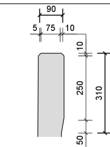
bovenrand rondom 1:10
