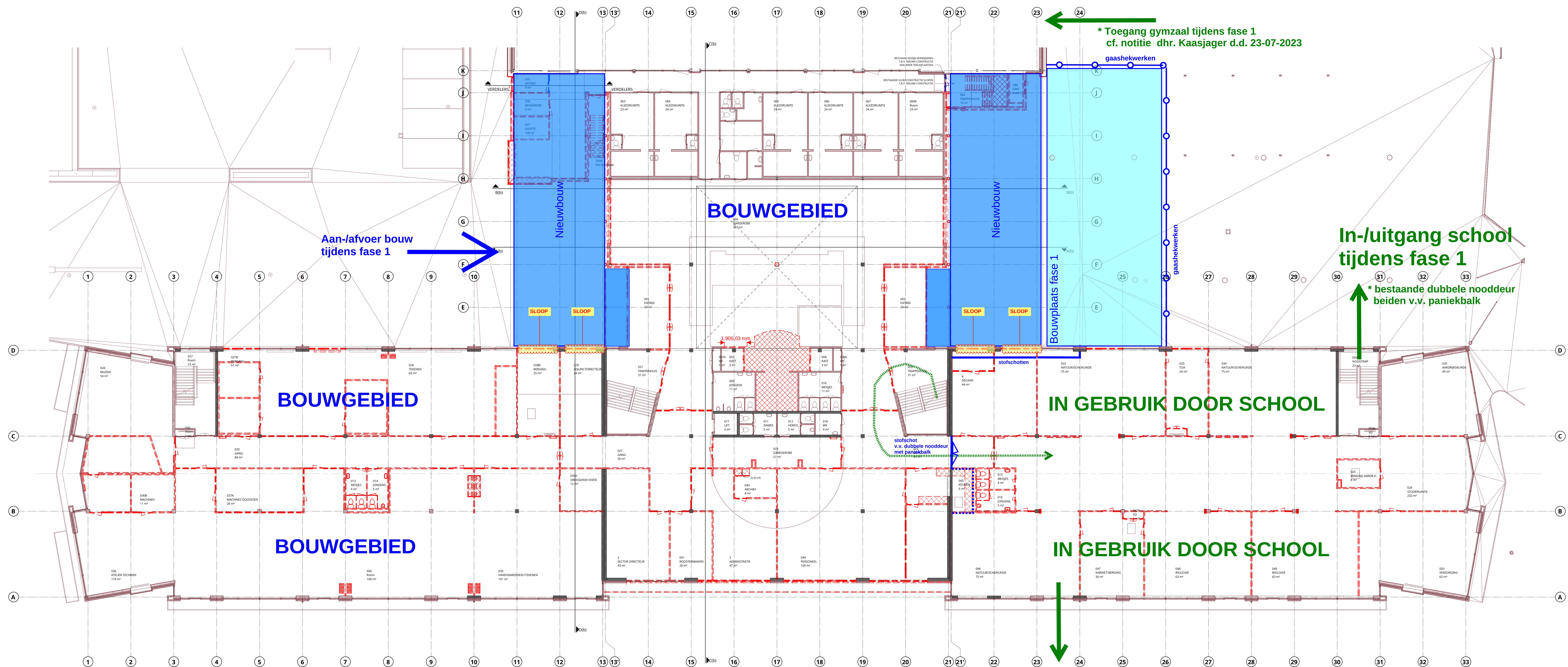
BEGANE GROND (bestaand) schaal 1:100
