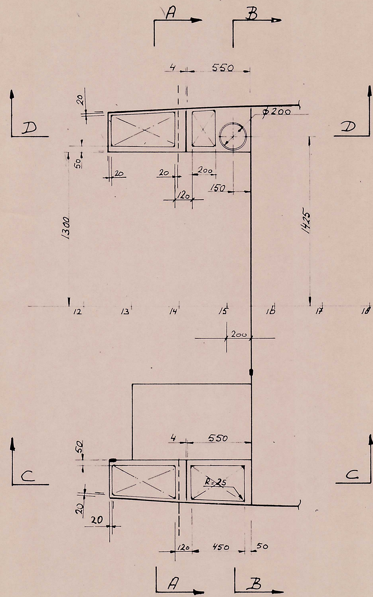
BOVEN AANZICHT DEK
