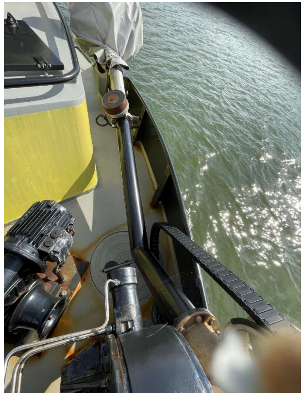
Uithouder met multibeam aan boord gedraait
