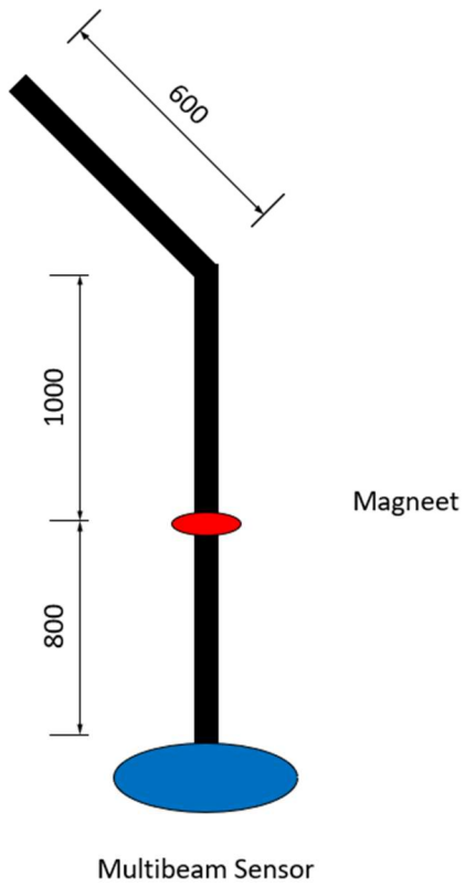
Hydrauliek TBV uithouder multibeam
