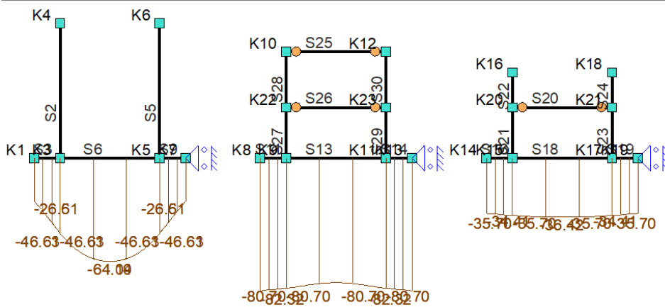
Fu.C.18 Gronddruk
