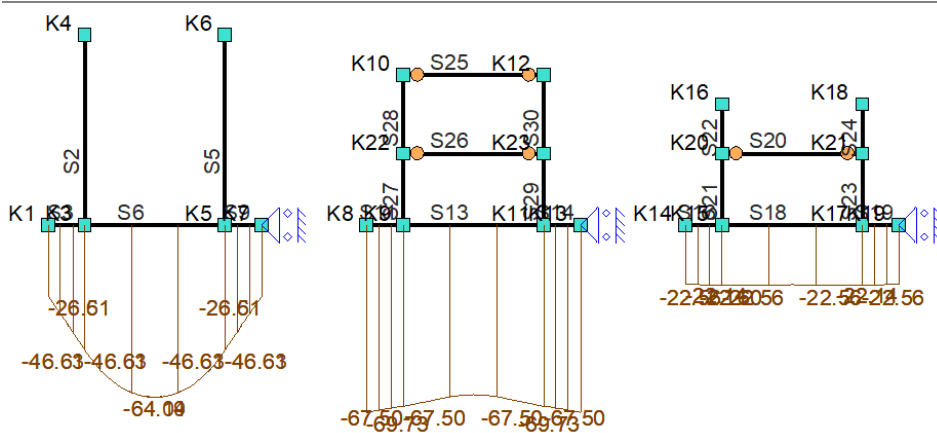
Fu.C.20 Gronddruk
