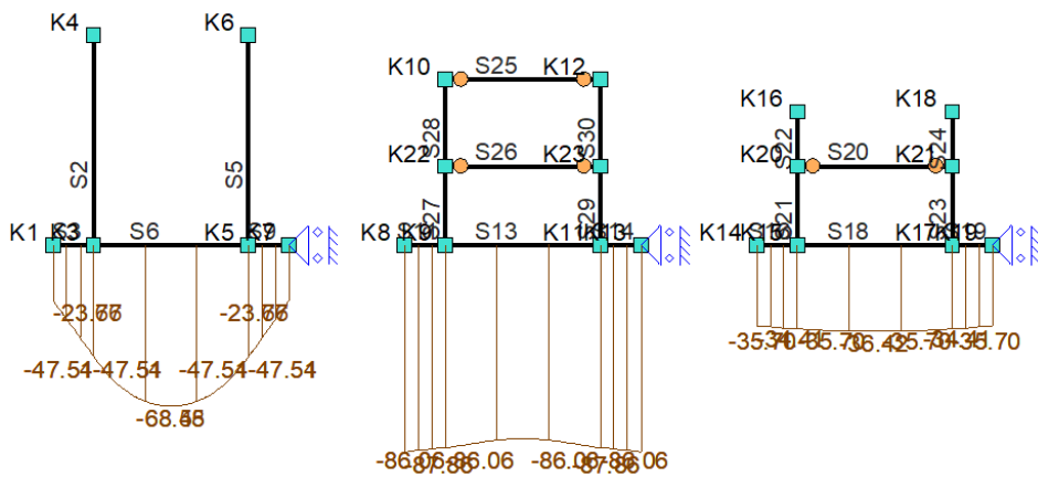
Fu.C.17 Gronddruk
