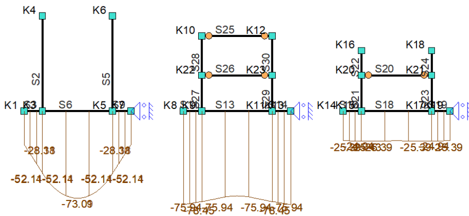
Fu.C.4 Gronddruk
