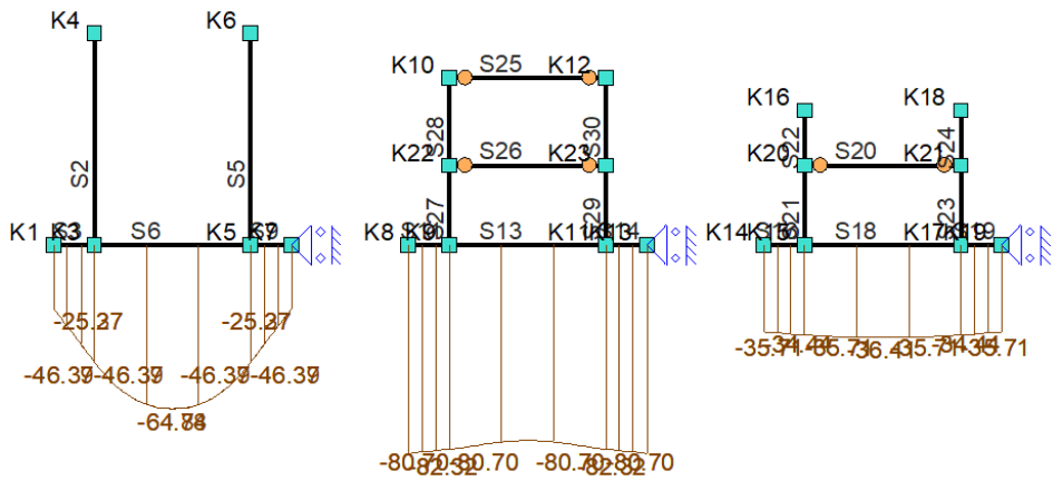
Fu.C.10 Gronddruk
