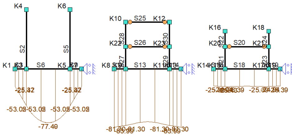
Fu.C.3 Gronddruk
