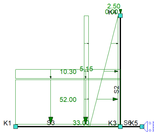
B.G.2: Gronddruk
