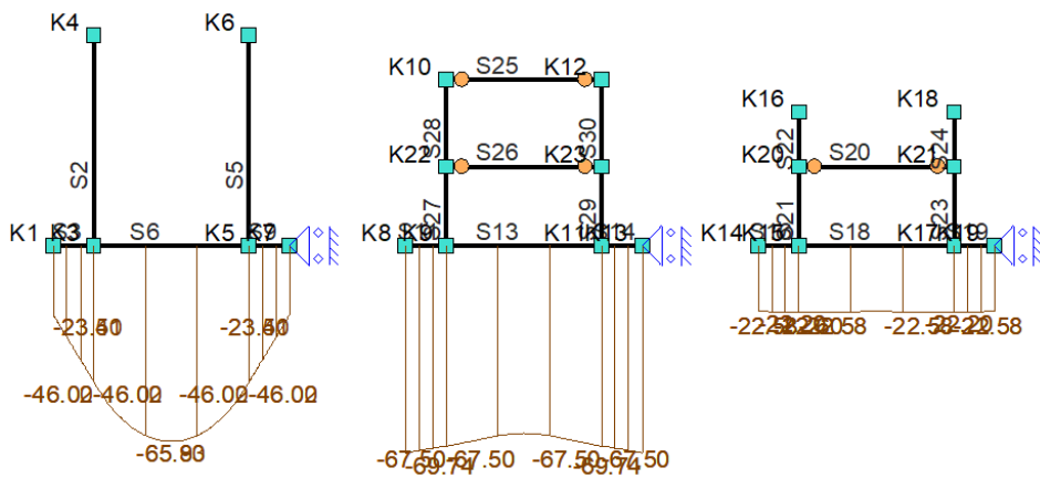
Fu.C.16 Gronddruk
