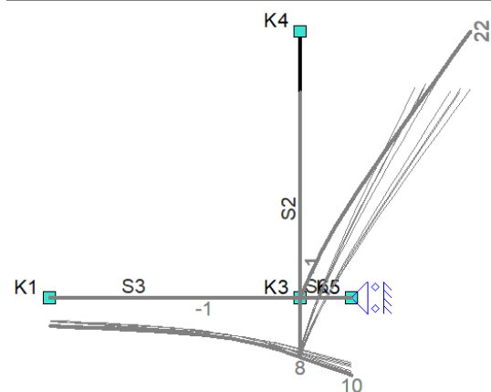
Ka.C. Omhullende Doorbuigingen
