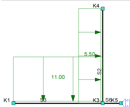
B.G.4: Verdeelde veranderlijke belasting
