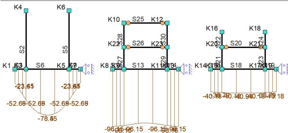
Fu.C.5 Gronddruk
