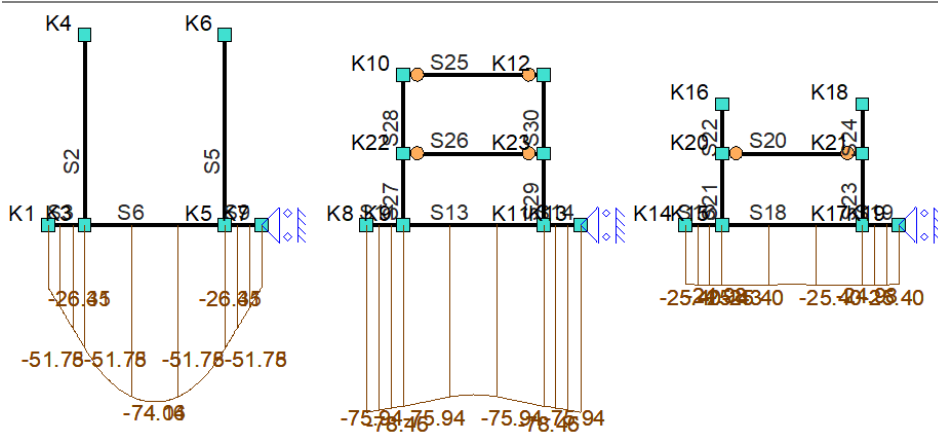
Fu.C.8 Gronddruk
