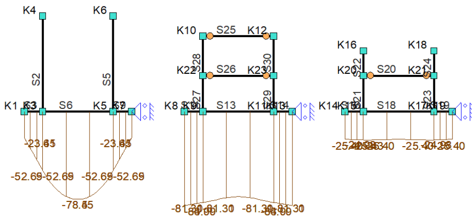
Fu.C.7 Gronddruk
