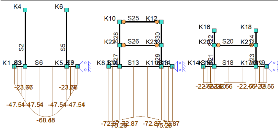
Fu.C.19 Gronddruk
