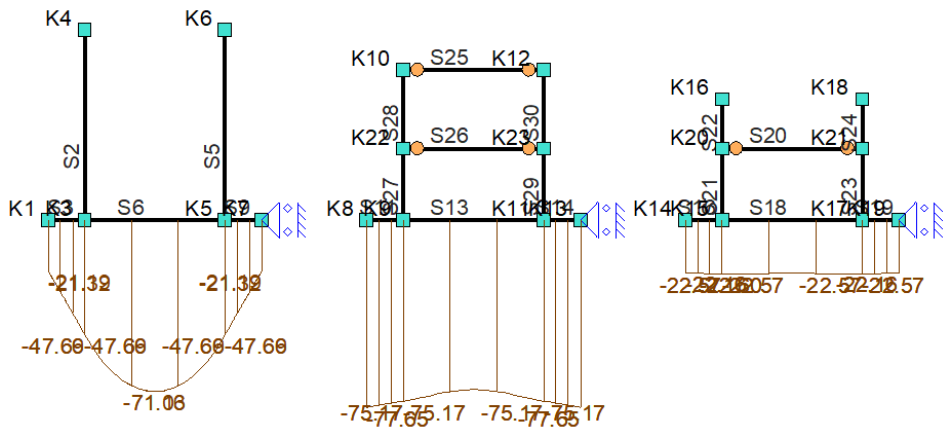
Fu.C.11 Gronddruk
