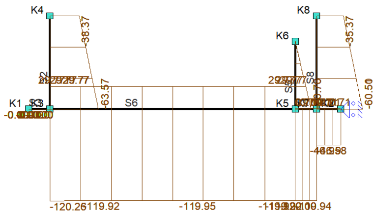
Fu.C. Omhullende Normaalkracht (Nx)
