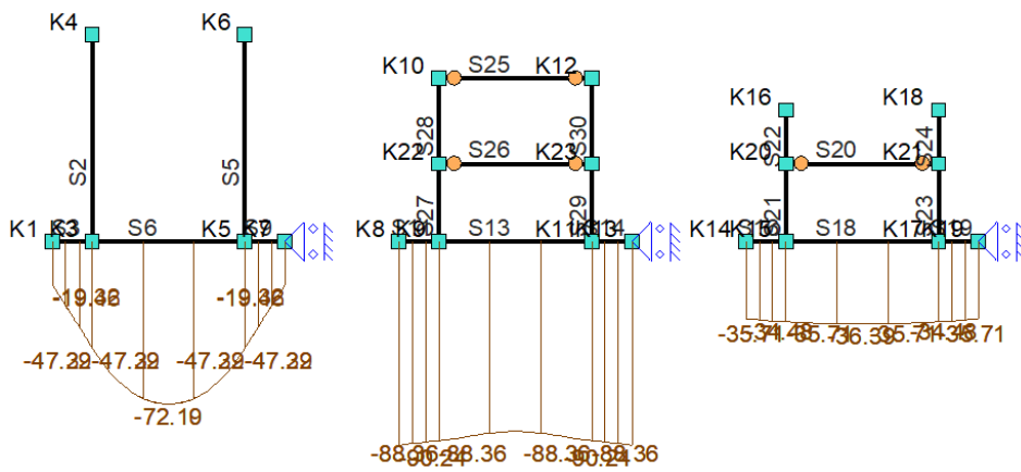
Fu.C.13 Gronddruk
