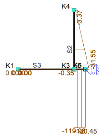
Fu.C. Omhullende Normalkracht (Nx)
