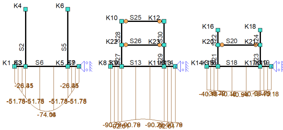
Fu.C.6 Gronddruk
