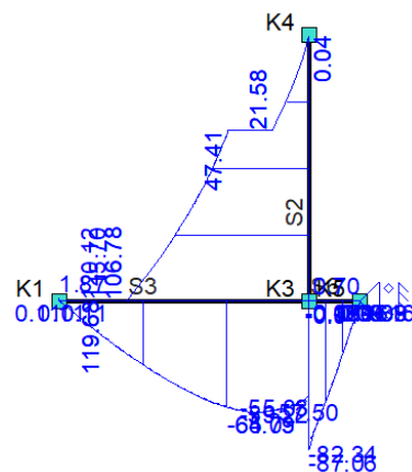
Fu.C. Omhullende Dwarskracht (Vz)
