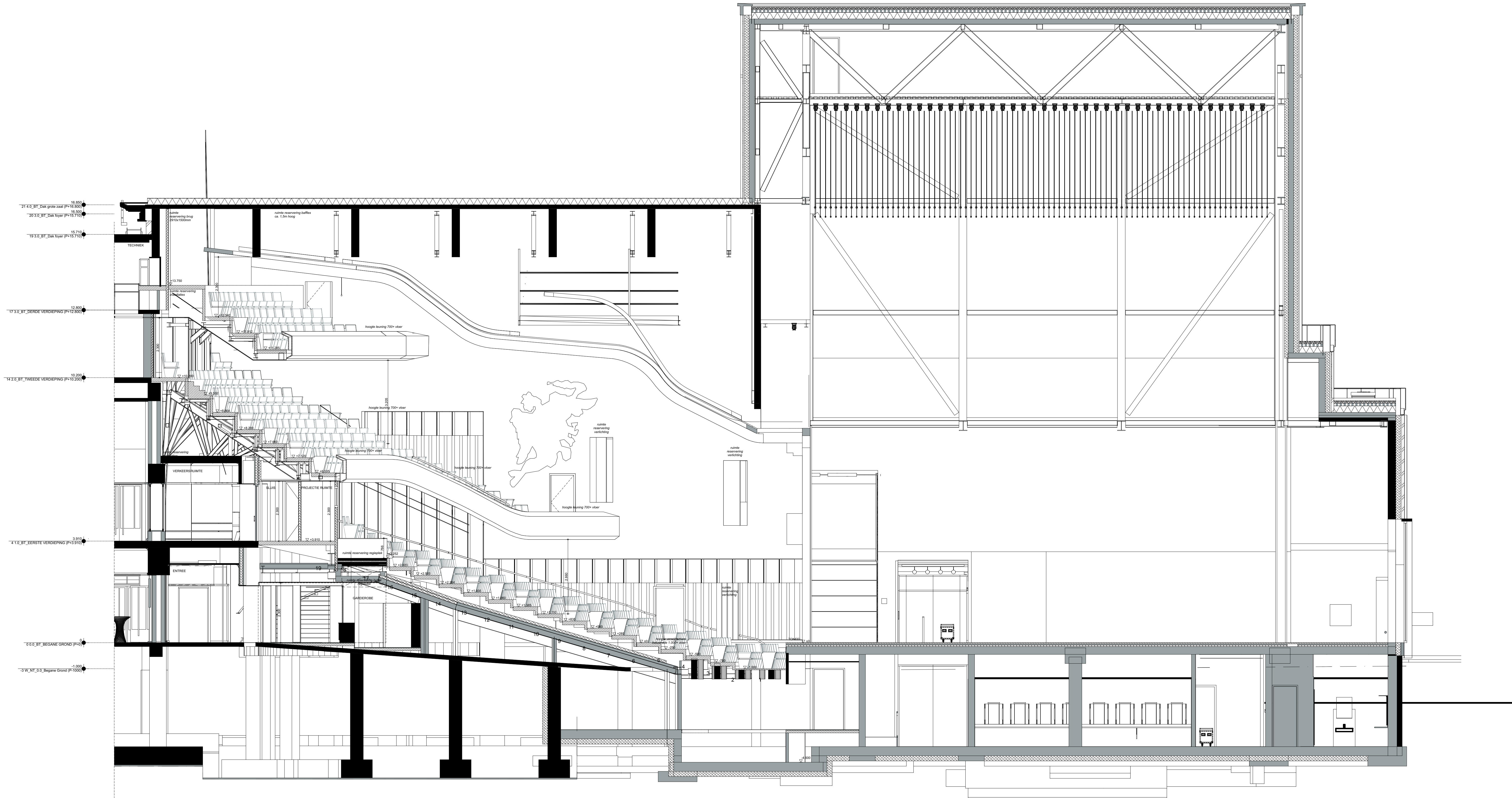
Langsdoorsnede
