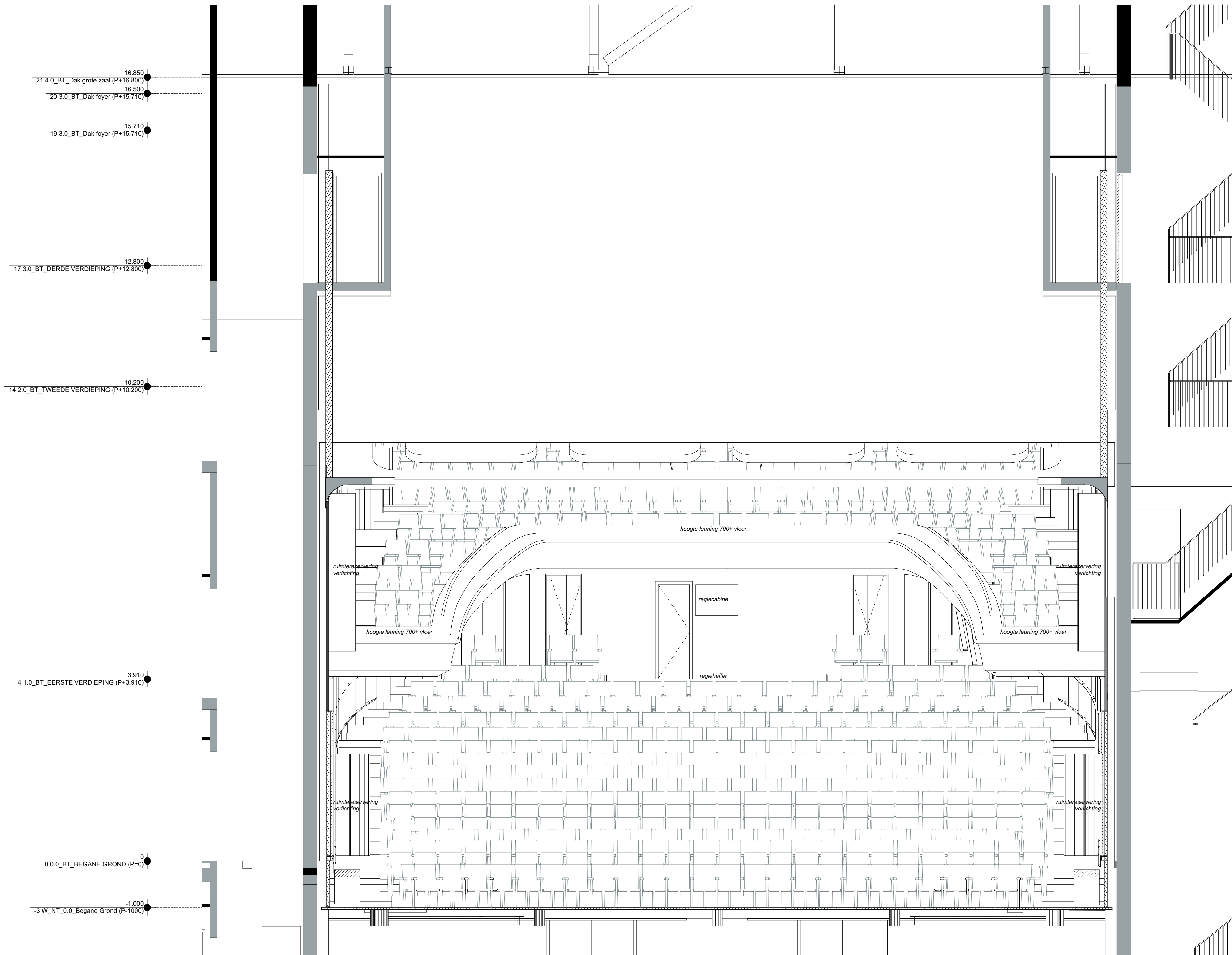
Dwarsdoorsnede
