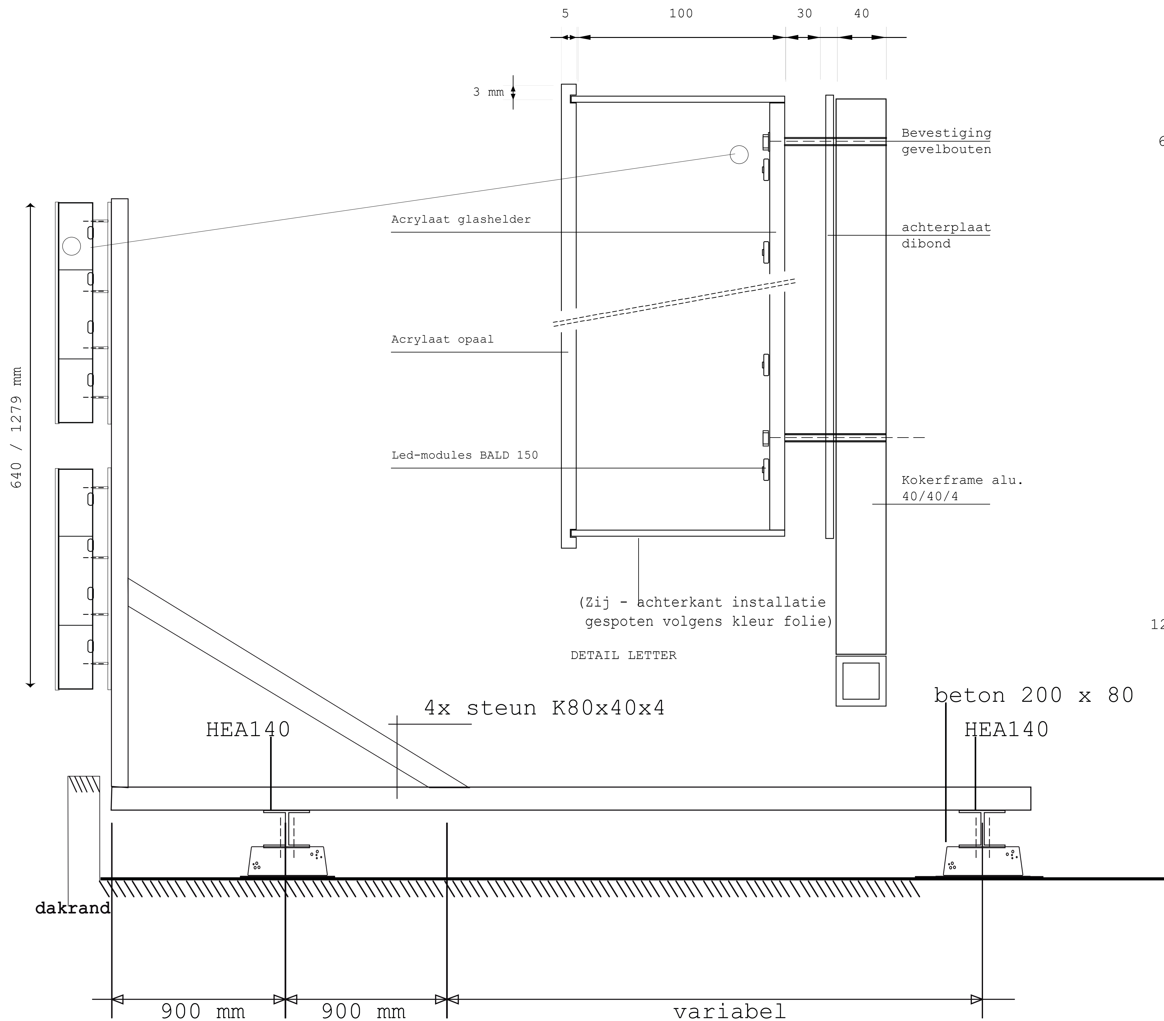
zijaanzicht Principe detail constructie LED-installatie
