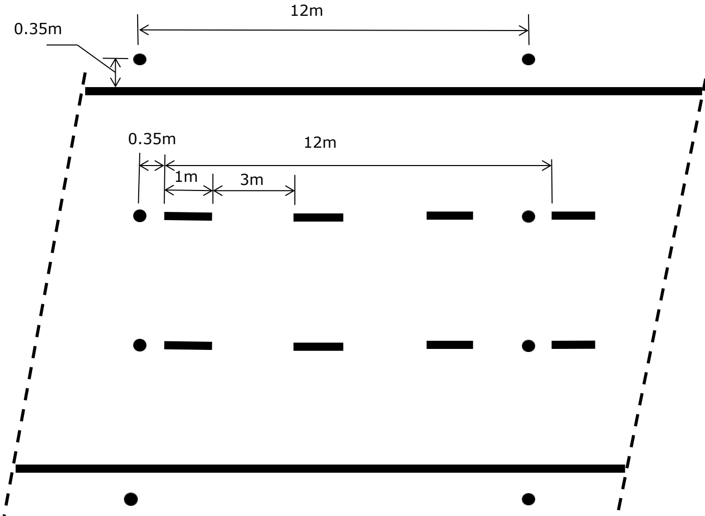
Figuur II; Schematische/niet op schaal getekende weergave van markeringsstippen in geval van een 1-3 streep
