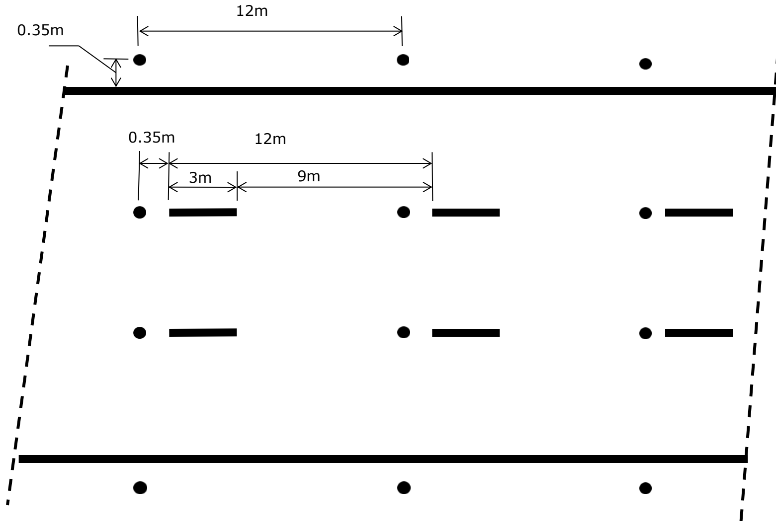
Figuur I; schematische/niet op schaal getekende weergave van markeringsstippen in geval van een 3-9 streep
