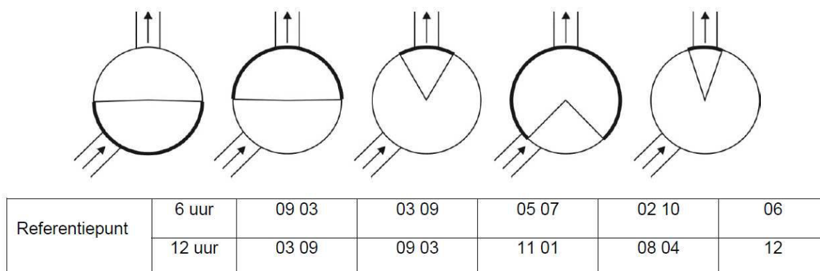
Figuur x: Voorbeelden van klokposities in rioolputten en inspectieputten (Figuur 4 uit NEN-EN 13508-2). In de bovenste rij is het referentiepunt (laagst gelegen uitgaande buis) 6 uur, in de onderste rij 12 uur.
