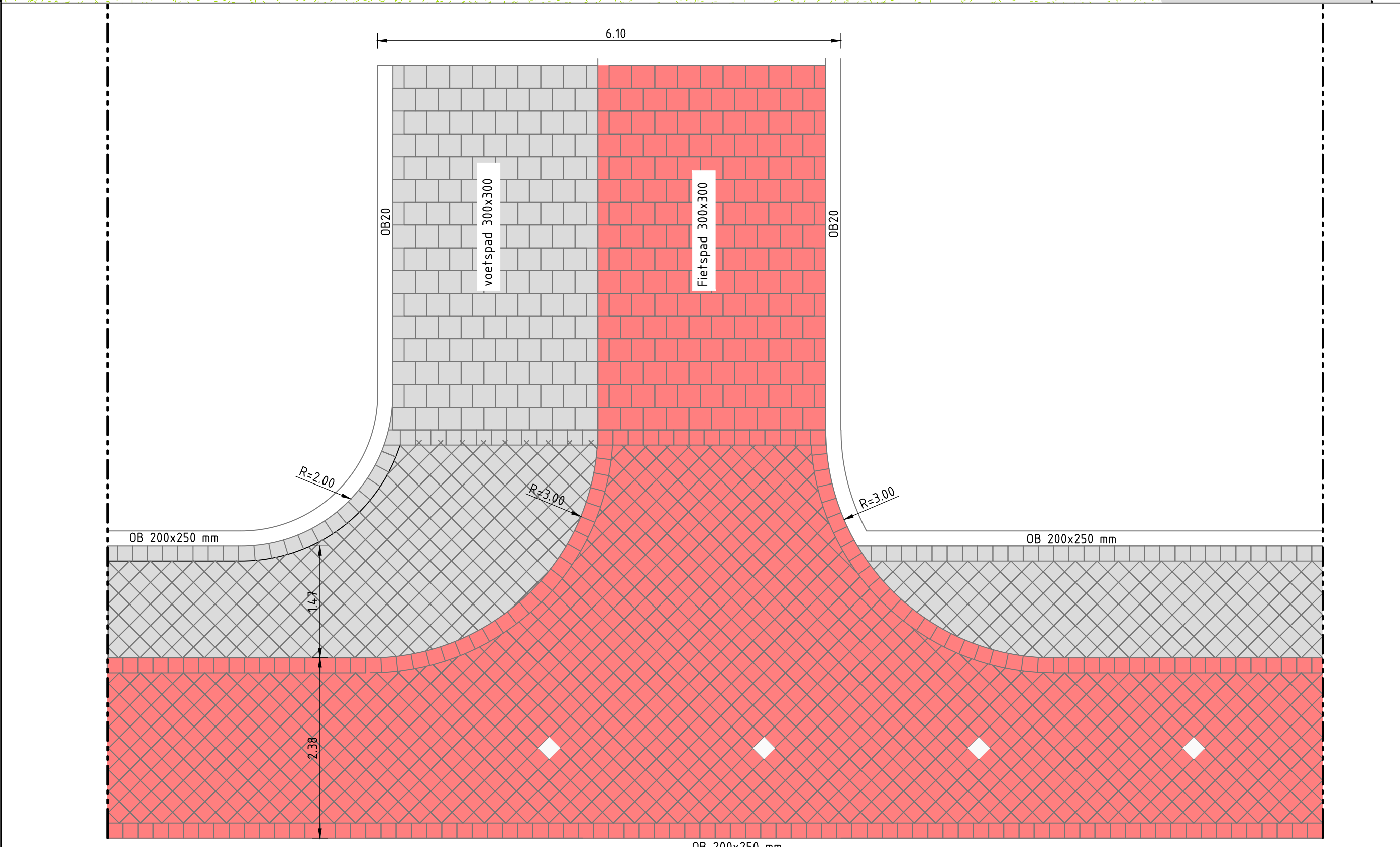
Detail 04: Aansluiting fietspad
