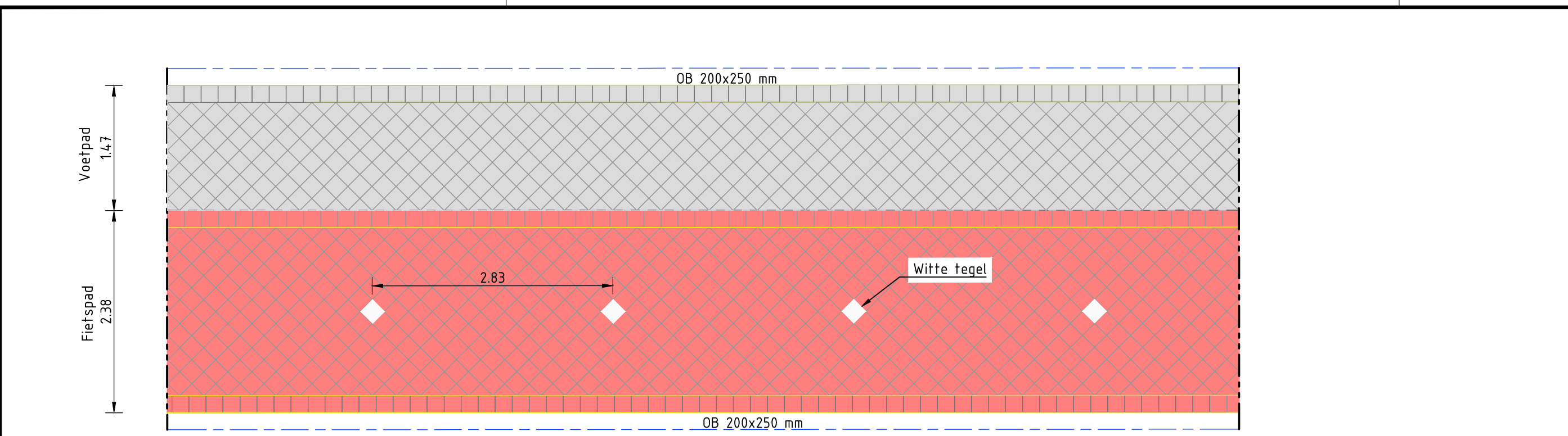
Detail 01: Diagonaalverband fiets-/voetpad
