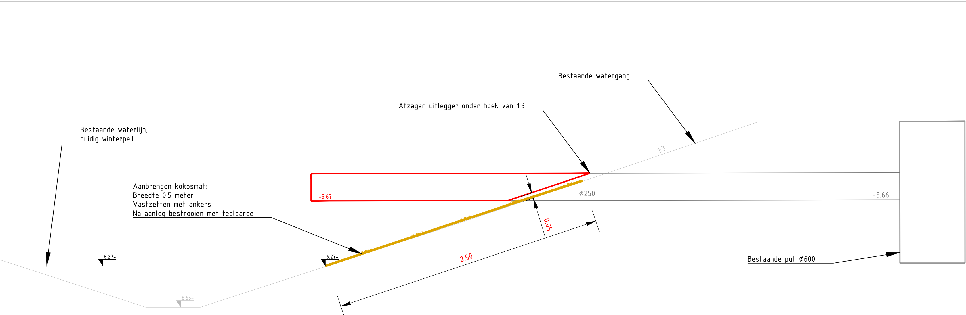
Detail 13: afwerken uitleggers SCHAAL 1 : 20
