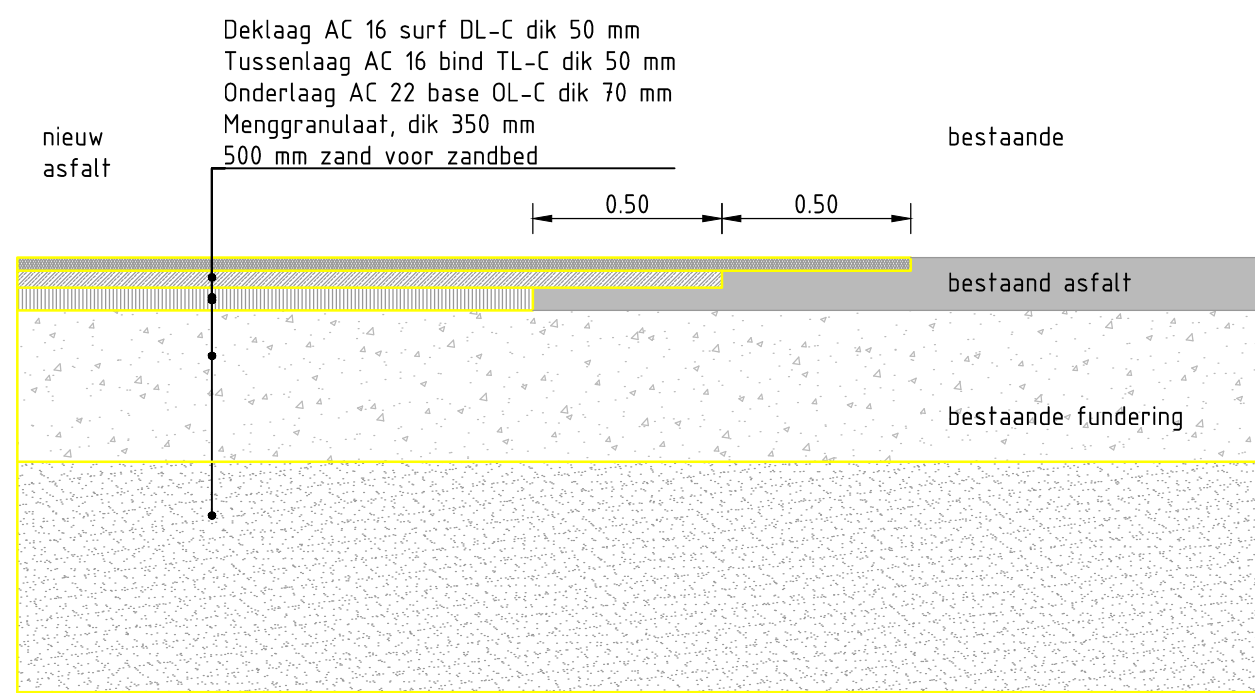
detail 11: doorsnede rijbaanaansluiting tijdens fasering schaal 1:20
