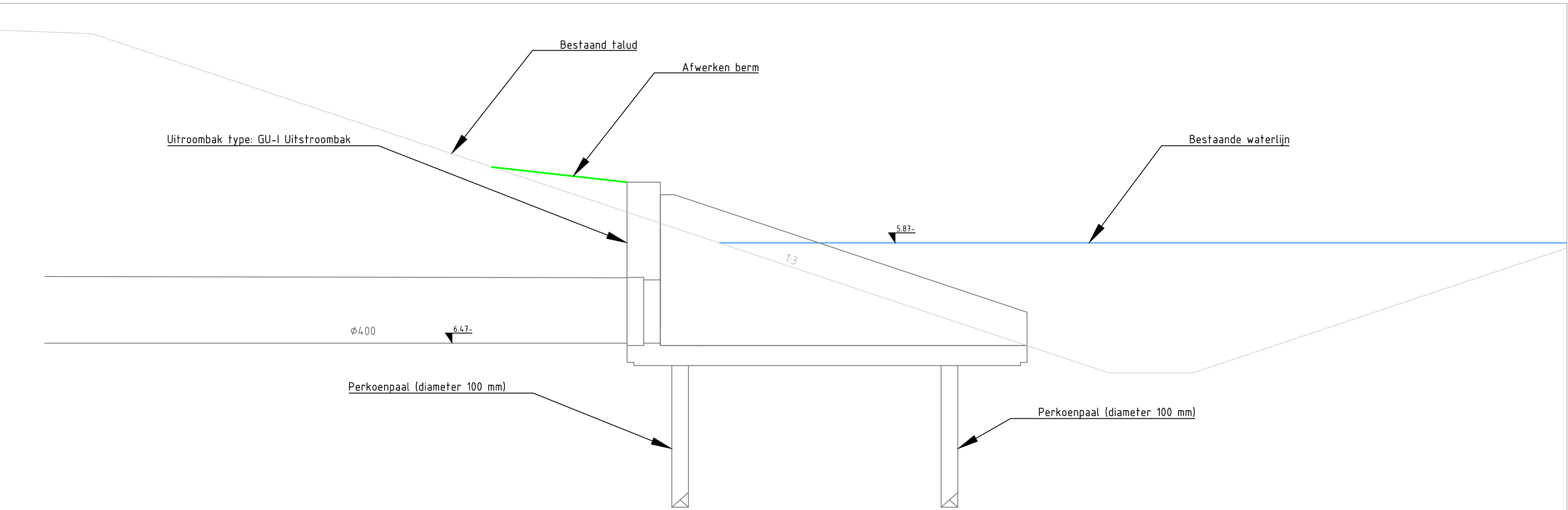
Detail 14: doorsnede uitroombak SCHAAL 1 : 20
