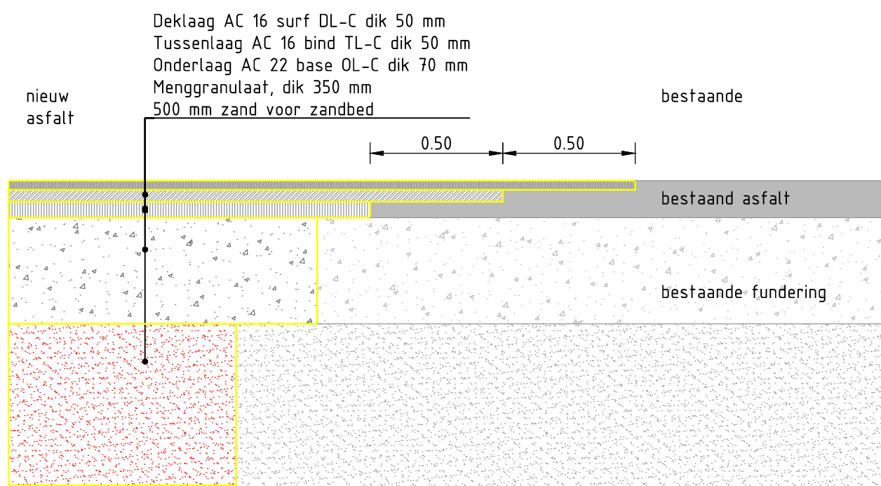
detail 10: doorsnede rijbaanaansluiting op bestaande situatie schaal 1:20
