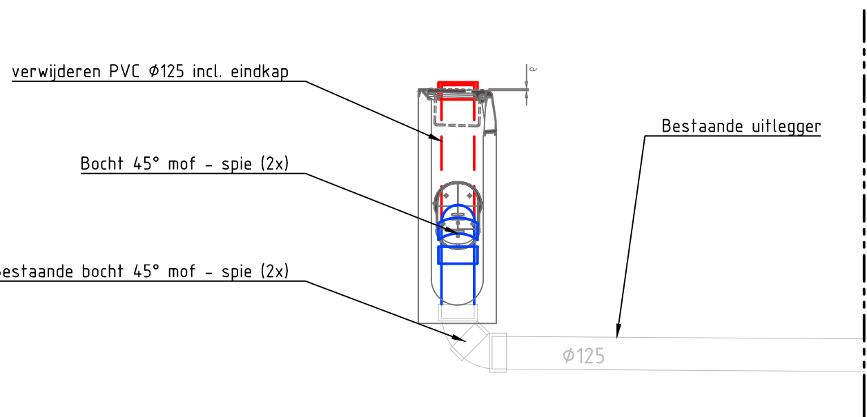
Principe detail 12: zijaanzicht kolkaansluiting schaal 1:20
