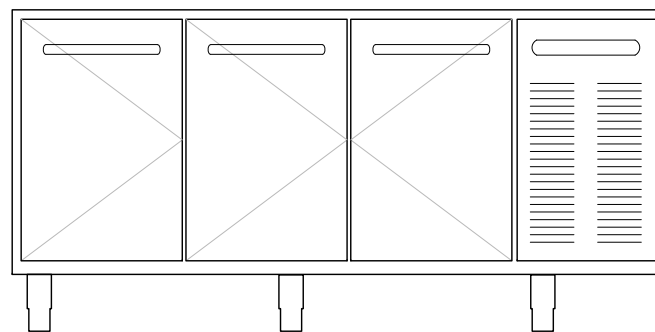
AA.09 Onderbouwkoeling 3 secties met iedere sectie een deur
