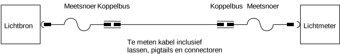
Figuur 2 Dampingmeting
