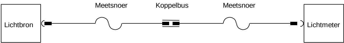
Figuur 1 Kalibreren meting (Lichtbron, Lichtmeter en meetsnoeren)
