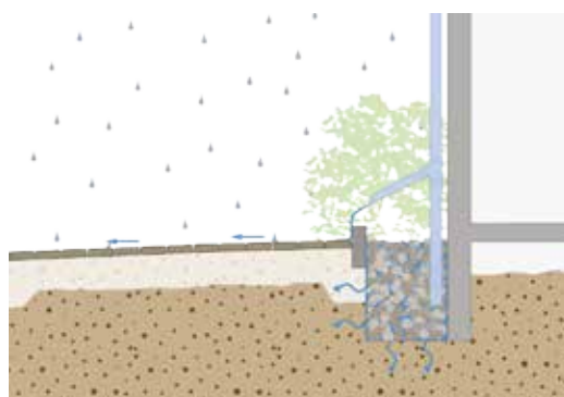
Schematische doorsnede van een geveltuin met grind en overstort naar de straat © Atelier GROENBLAUW
