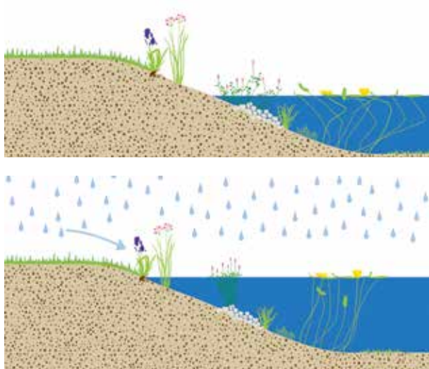
Schematische doorsnede van een regenwaterbuffervijver © Atelier GROENBLAUW
