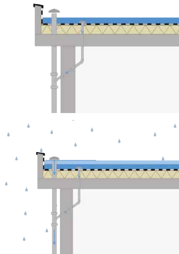
Schematische doorsnede van een regendak bij een normale en een extreme regenbui © Atelier GROENBLAUW
