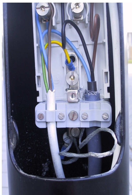
4. Grondkabel en armatuursnoer onder trekontlasting vastzetten.
