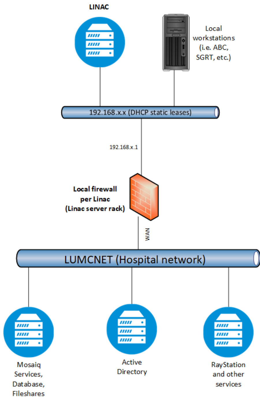
Firewall Overzicht LUMC
