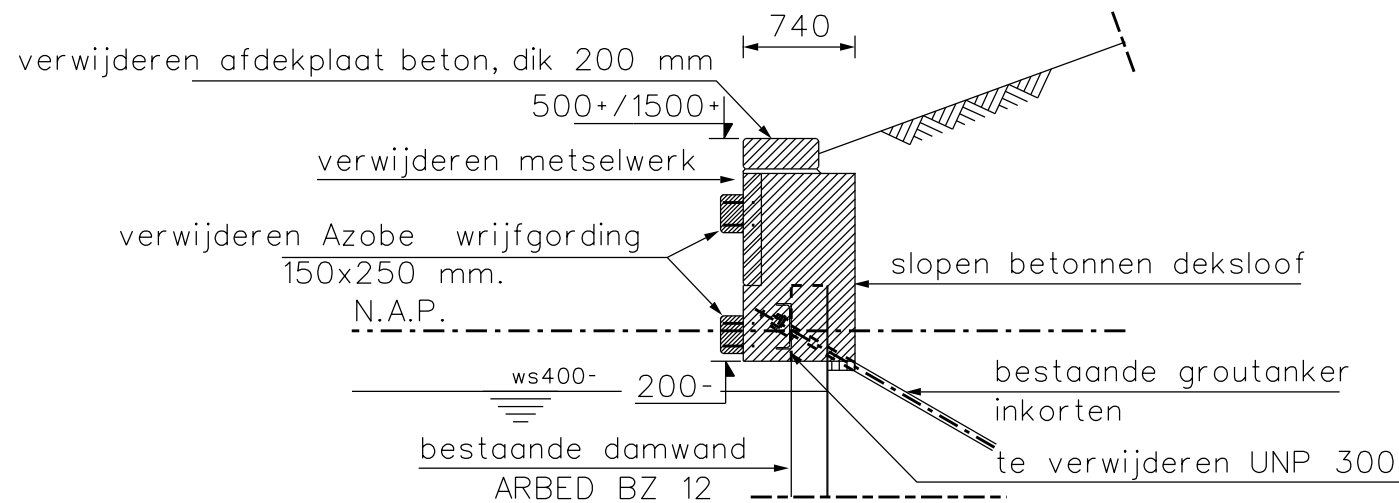
Doorsnede A (1:50)
