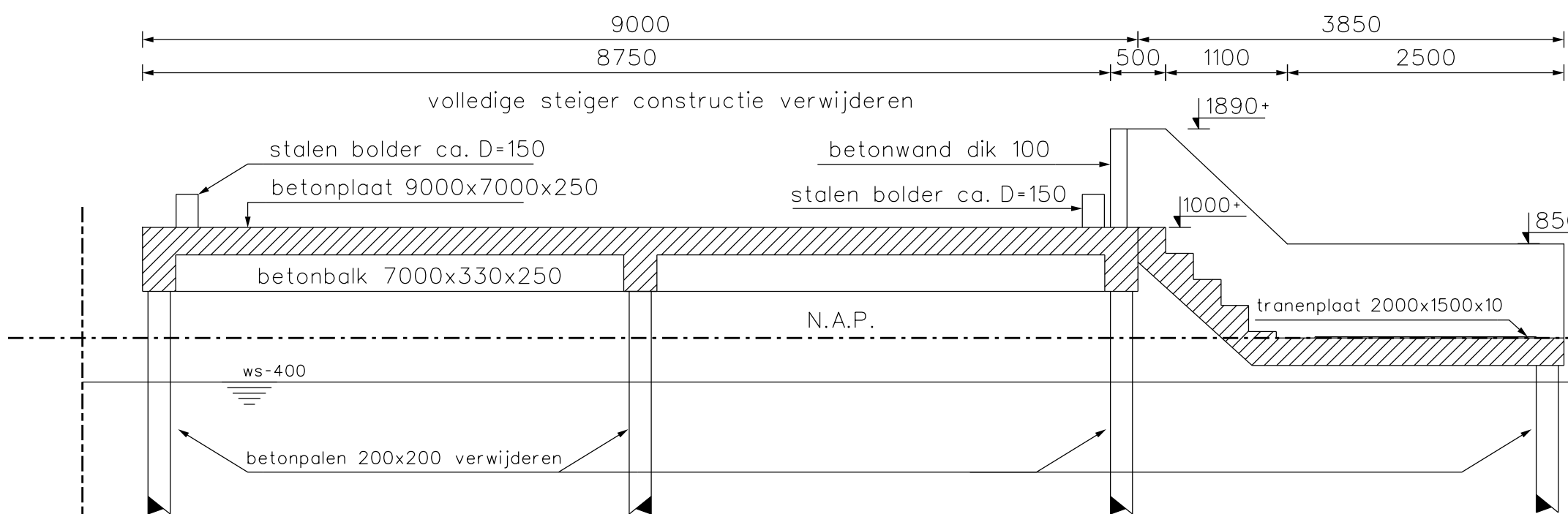
Doorsnede D (1:50)
