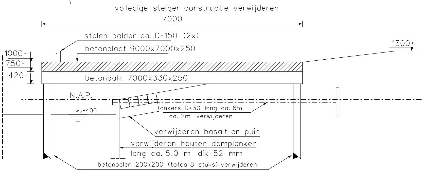
Doorsnede C (1:50)
