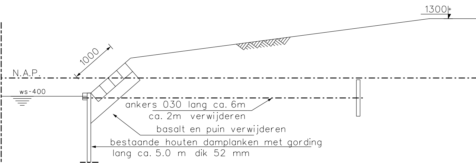
Doorsnede B (1:50)
