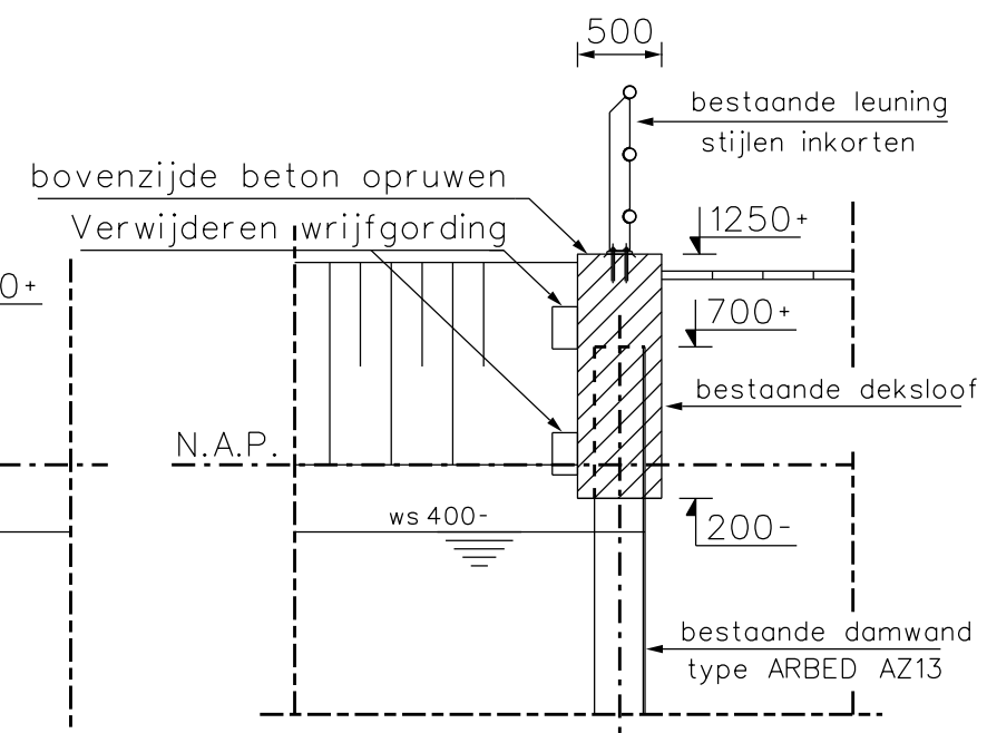
Doorsnede E (1:50)
