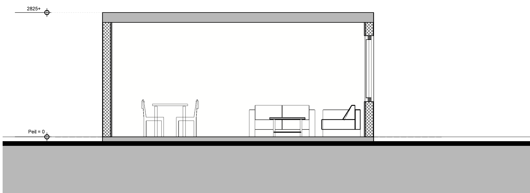
DWARSDOORSNEDE
