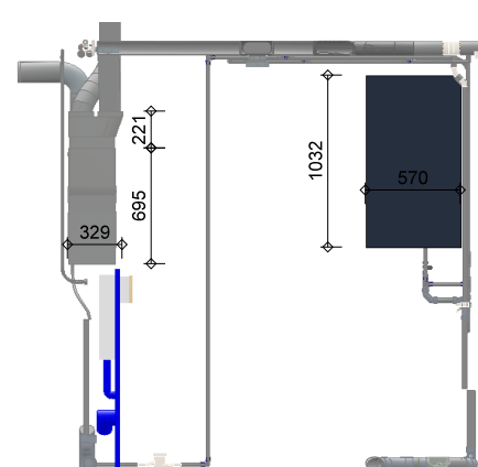
ZIJAANZICHT
