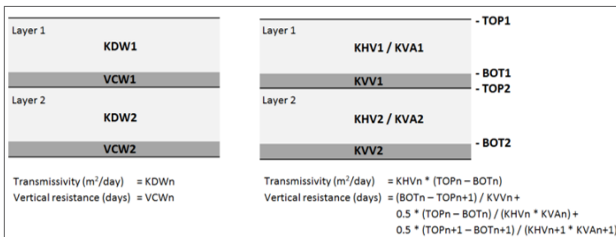
Figuur 2: Verschil in schematisatie lagenmodel Triwaco/flairs (links) en MODFLOW-2005 (rechts) (Bron figuur: iMod handleiding)
