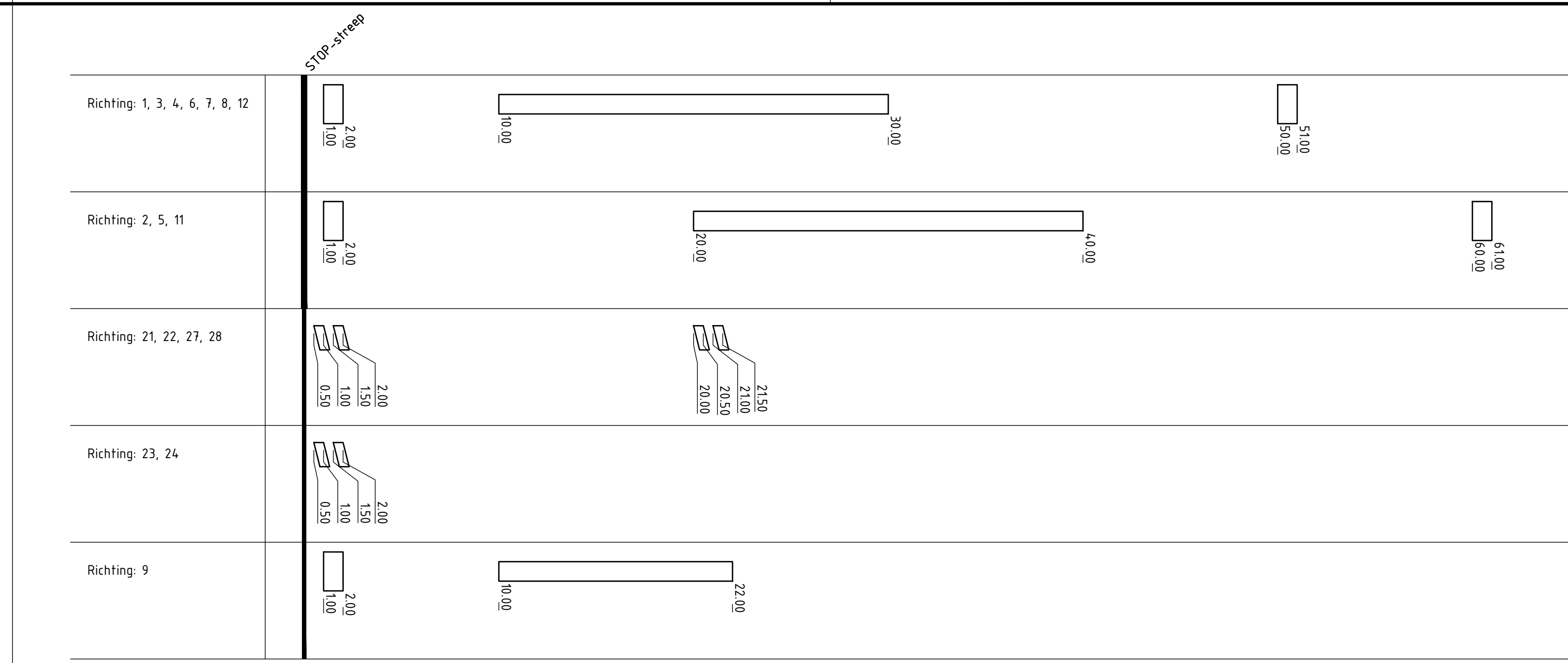
Detectielussenschema
