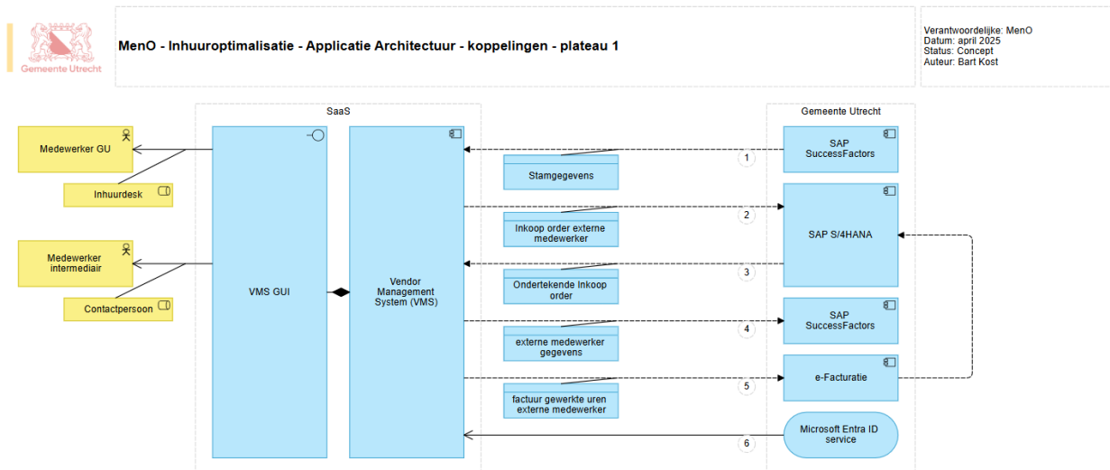
Figuur 1: Applicatie Architectuur
