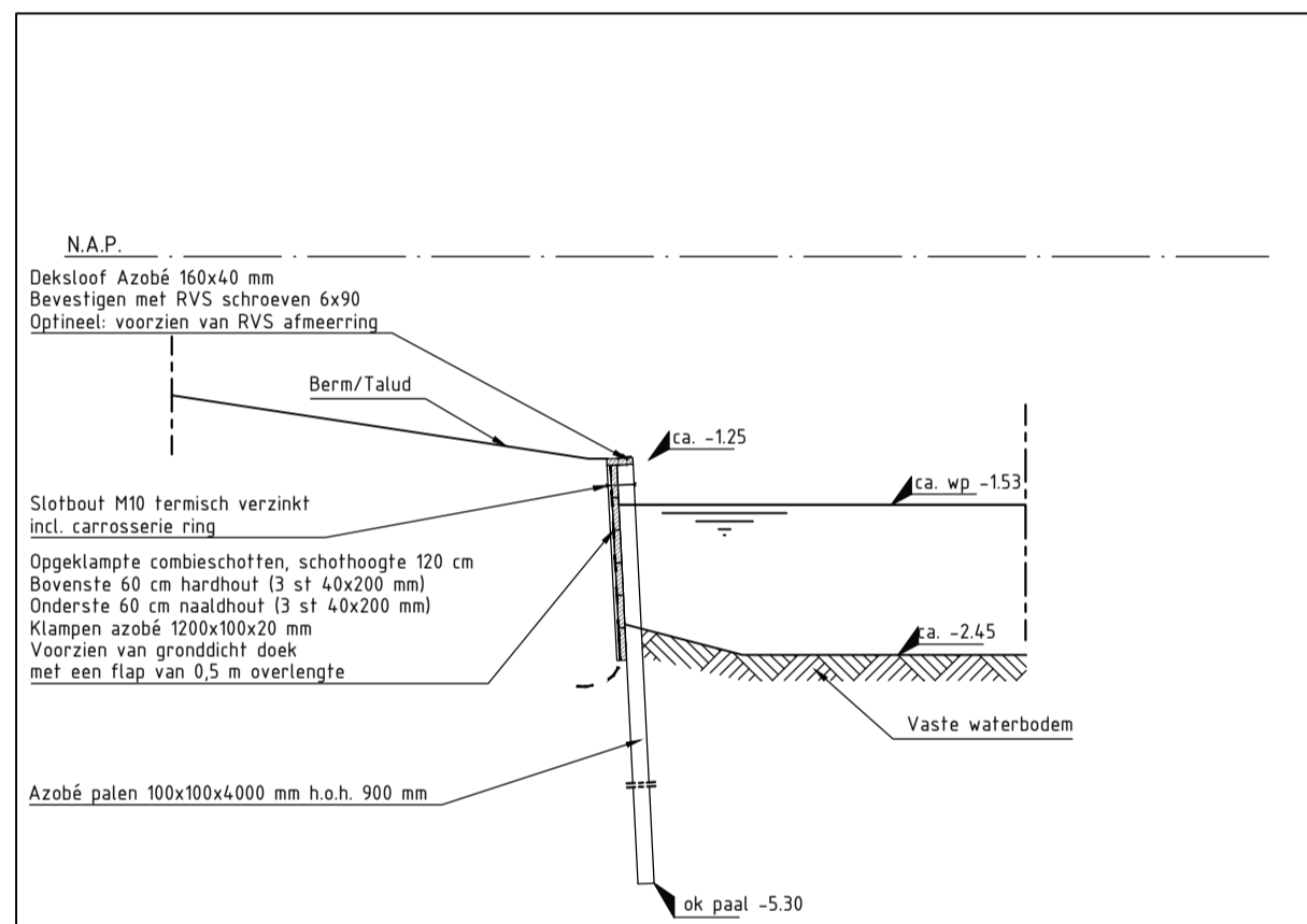
Principedetail opgeklampt schot hardhout / naaldhout Hoogte ca. 100 cm kerend Schaal 150
