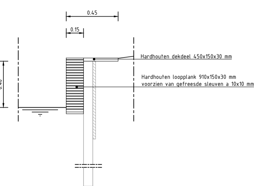
Detail: Zij aanzicht faunatrapp HIP Groen tot 400mm Schaal 120
