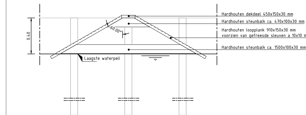
Detail: Vooraanzicht faunatrapp HIP Groen tot 400mm Schaal 120
