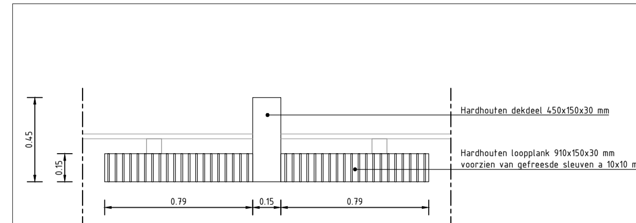
Detail: Bovenaanzicht faunatrapp HIP Groen tot 400mm Schaal 120
