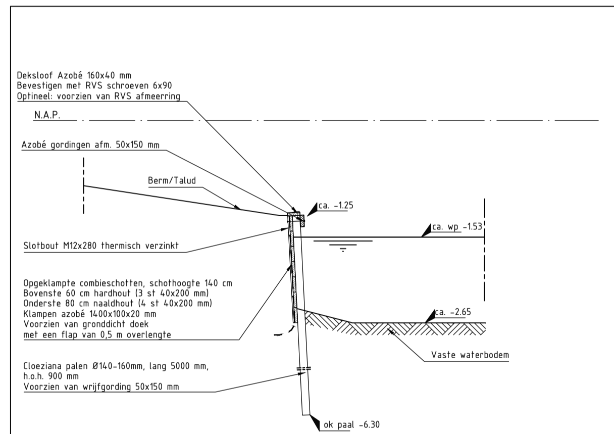
Principedetail opgeklampt schot hardhout / naaldhout Hoogte ca. 120 cm kerend (locatie: Rozendaal) Schaal 150
