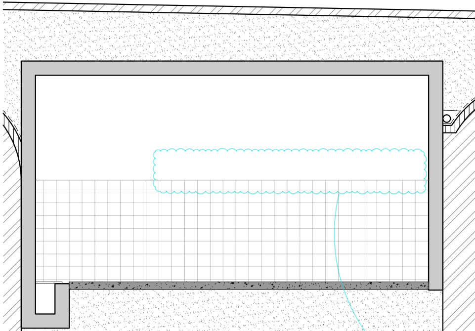
Doorsnede A
