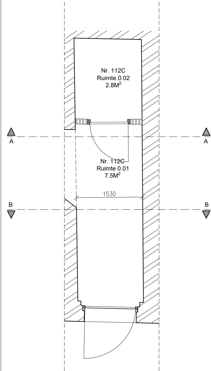
Plattegrond
