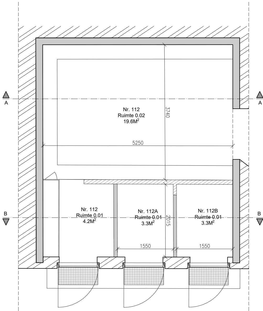
Plattegrond
