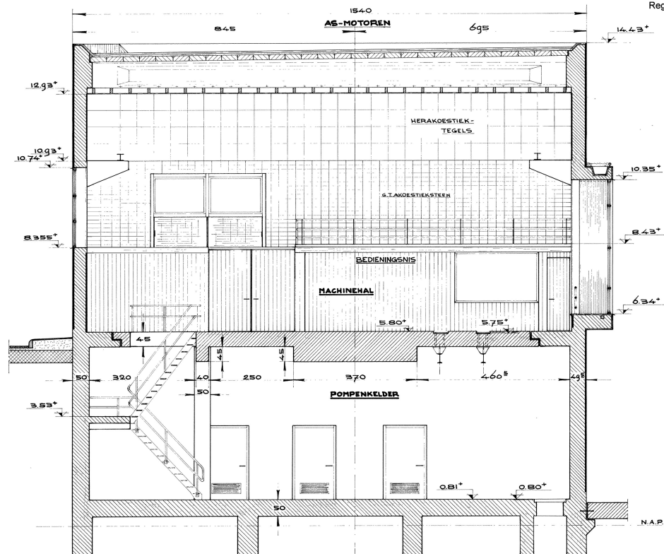
DOORSNEDE D-D
