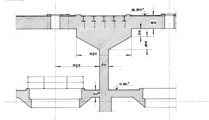
DOORSNEDE OVER AS-MOTOREN
