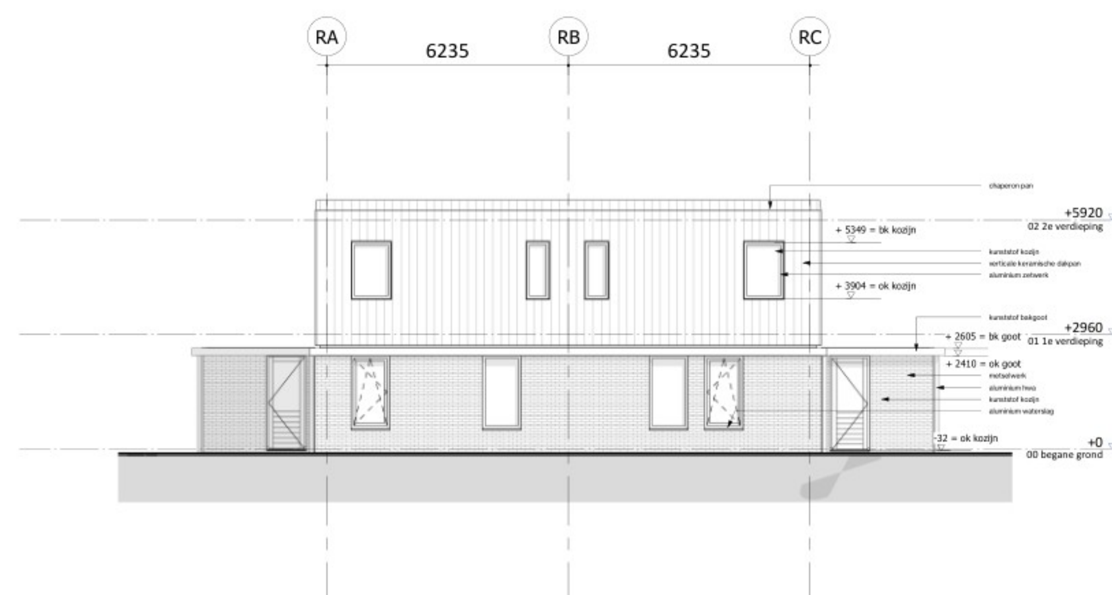
Achtergevel (Noordgevel)
