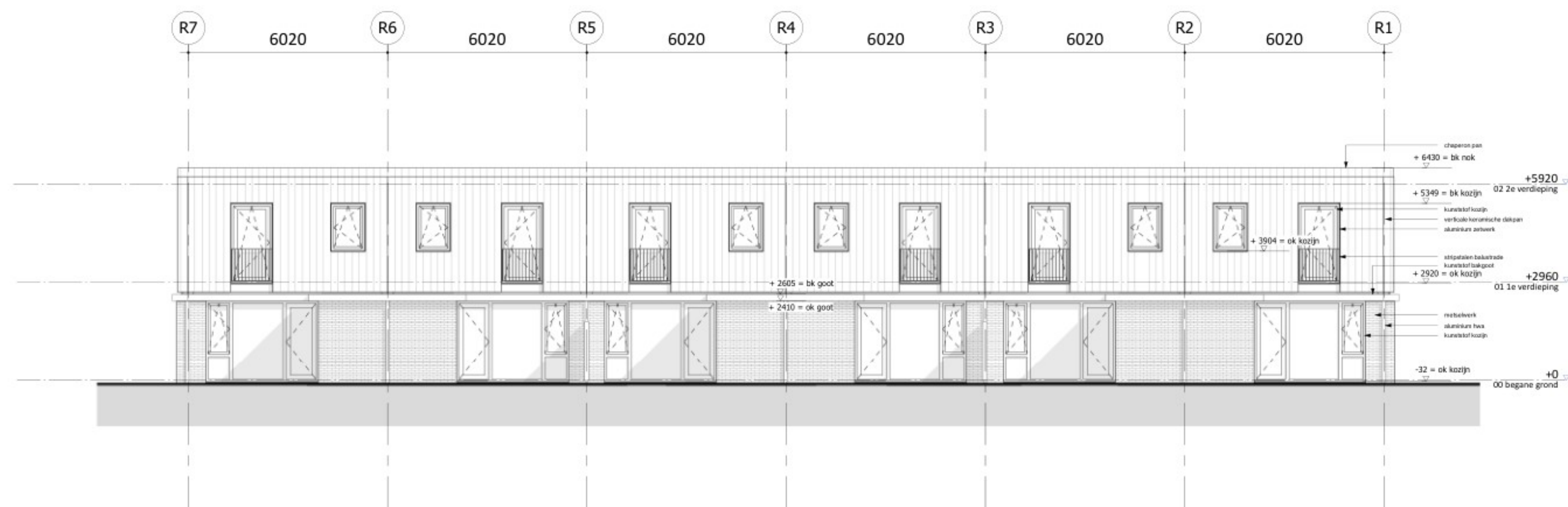
Linkerzijgevel (Westgevel)
