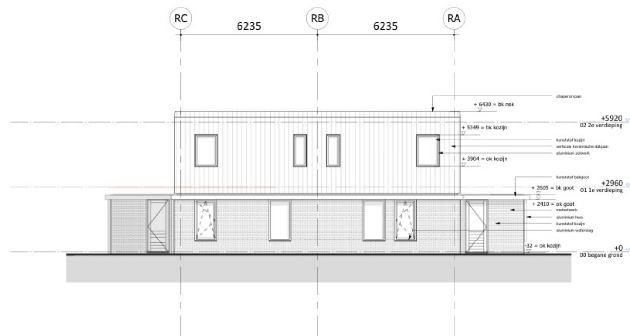
Voorgevel (Zuidgevel)
