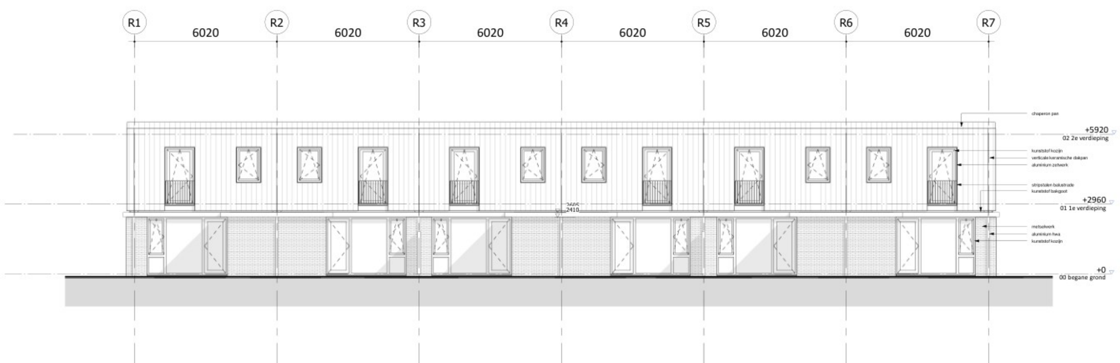
Rechterzijgevel (Oostgevel)
