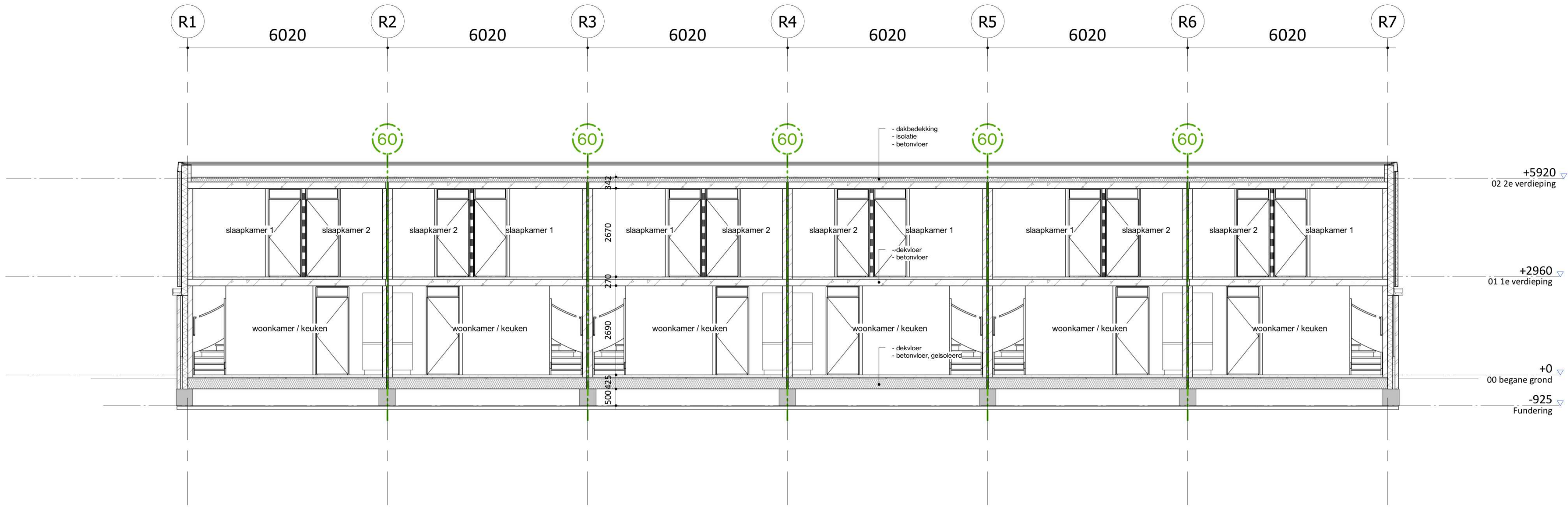
Doorsnede A
