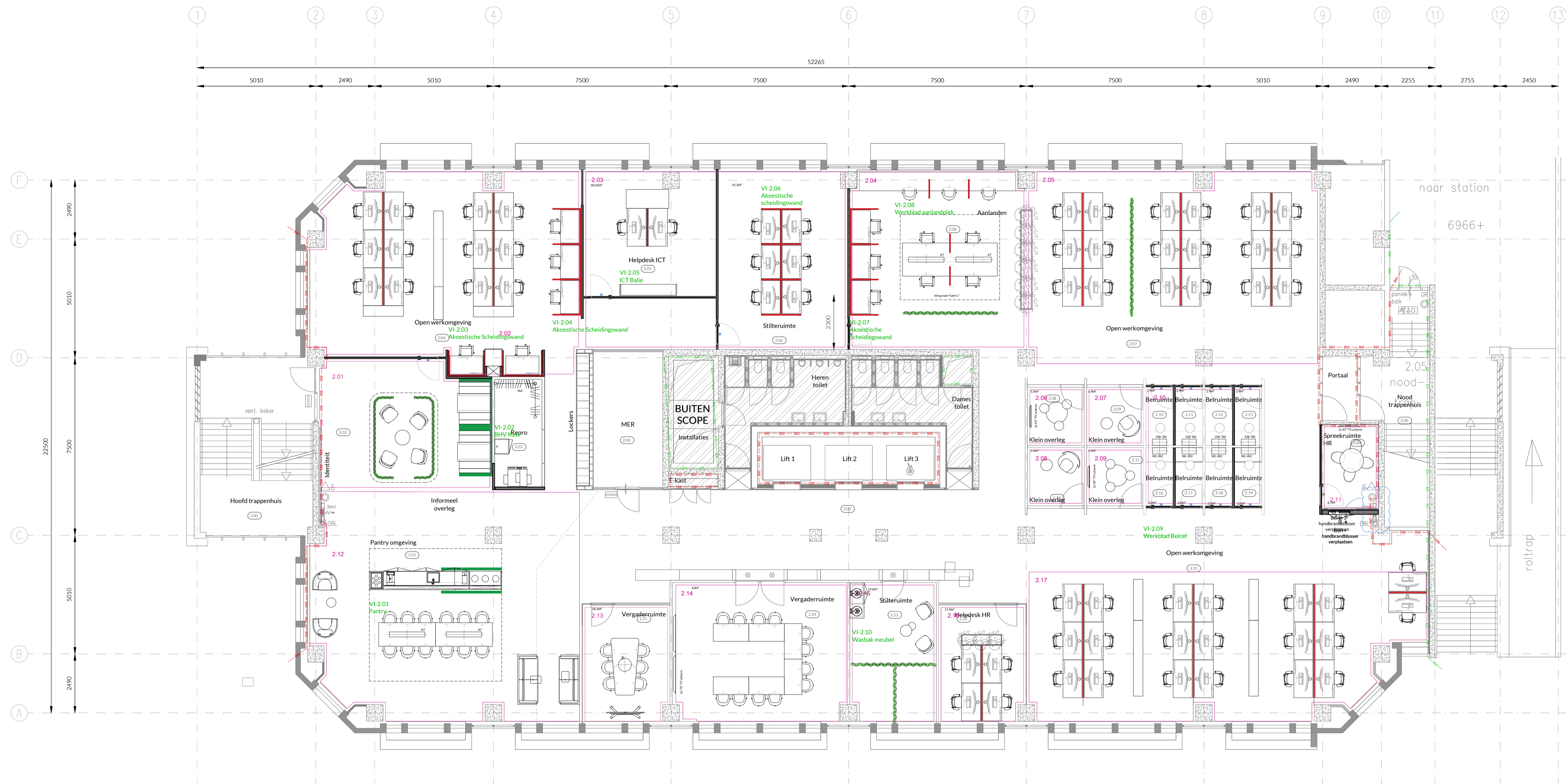
2e verdieping | 8.460+P
