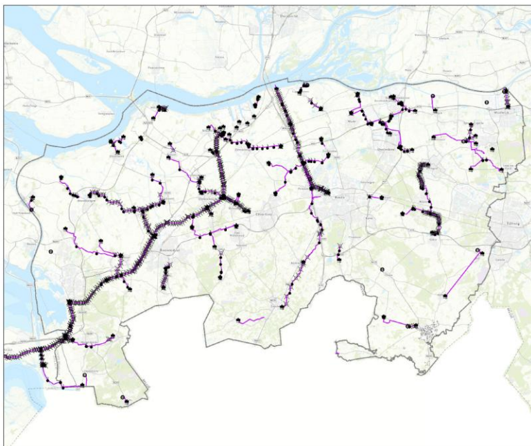
Persleidingareaal WBD met RWZI's, RG's, ontluchters, afsluiters en mangaten.
