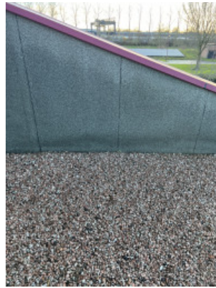
Plooi vorming in opstand
