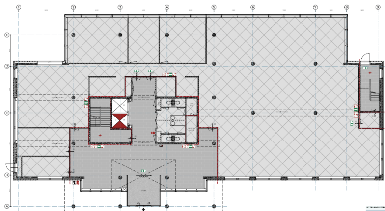
Figuur 4. Plattegrond begane grondlaag
